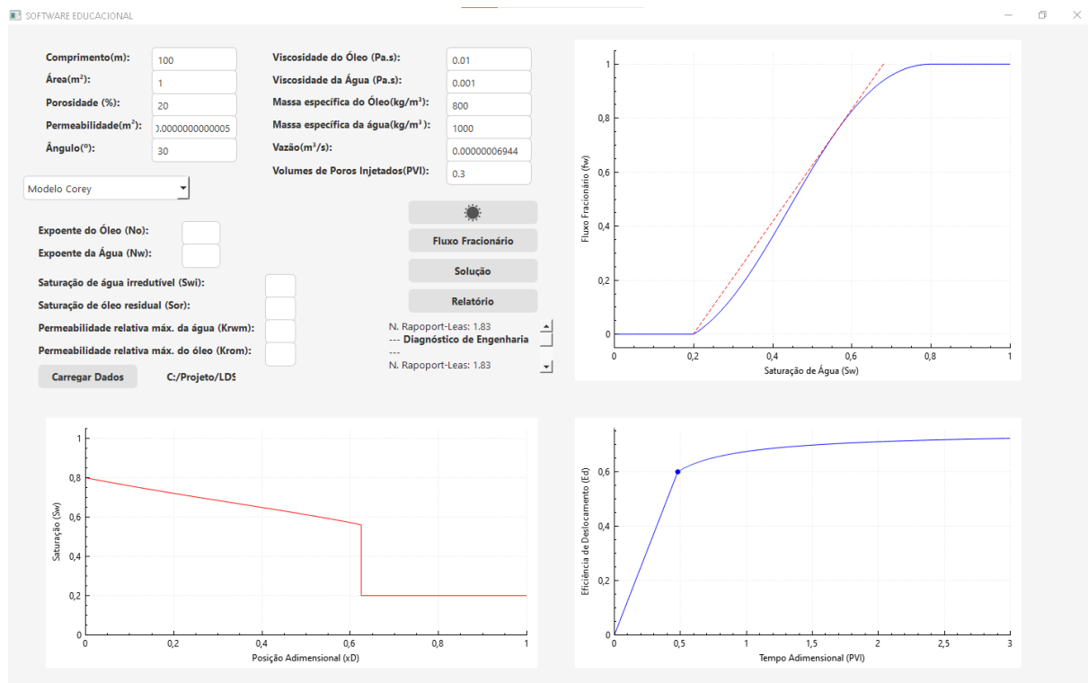
Figura 8.29: Tela do programa exibindo o perfil de saturação retardado para injeção ascendente em active ( \alpha = 30^\circ )
