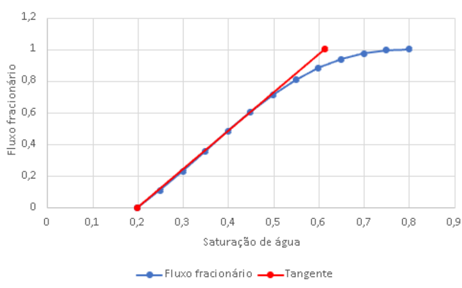
Figura 8.24: Gráfico analítico do fluxo fracionário e da tangente de Welge computados em planilha discreta para o modelo de Corey (Teste 2, Cenário A)
