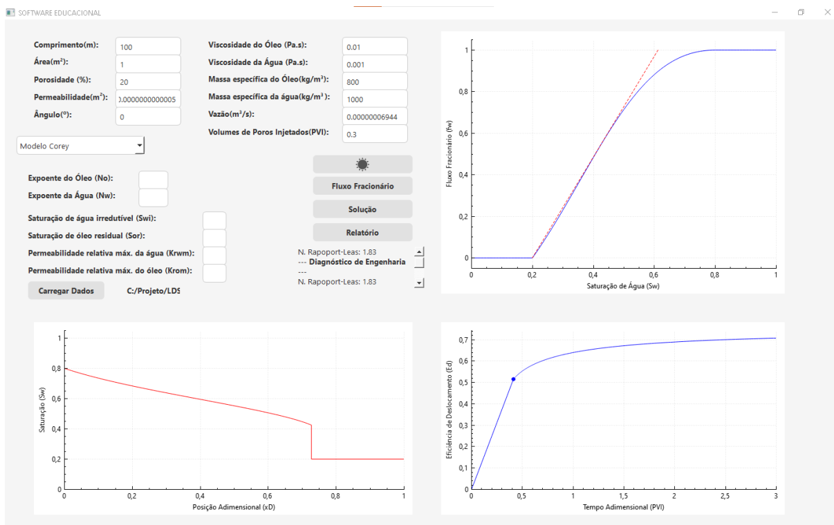
Figura 8.20: Tela do programa exibindo o perfil de saturação e a eficiência de deslocamento para injeção em reservatório horizontal ( \alpha = 0^\circ )
