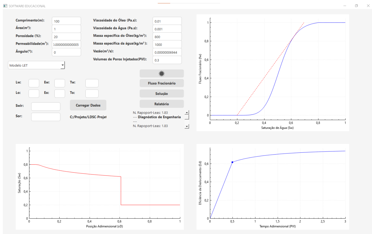
Figura 8.30: Painel principal do simulador processando o escoamento governado pelas curvas de permeabilidade do modelo LET
