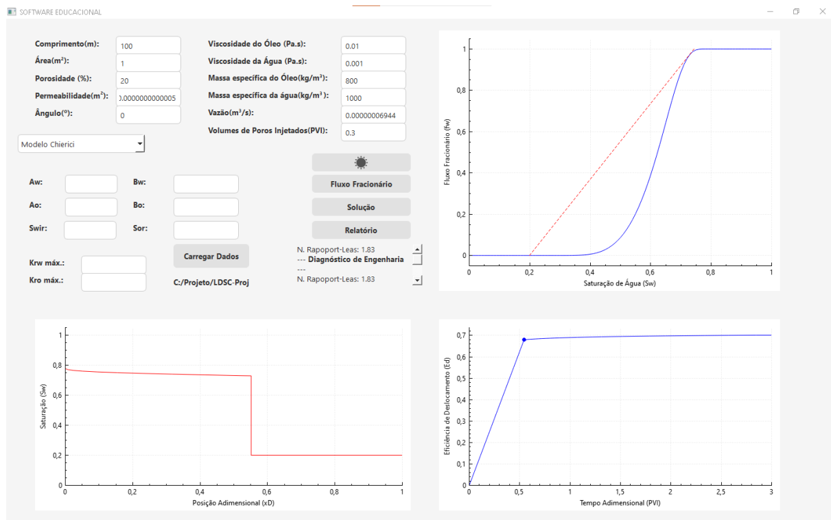
Figura 8.33: Pannel de resultados da interface gráfica demonstrando a estabilidade computacional na interpolação do modelo de Chierici
