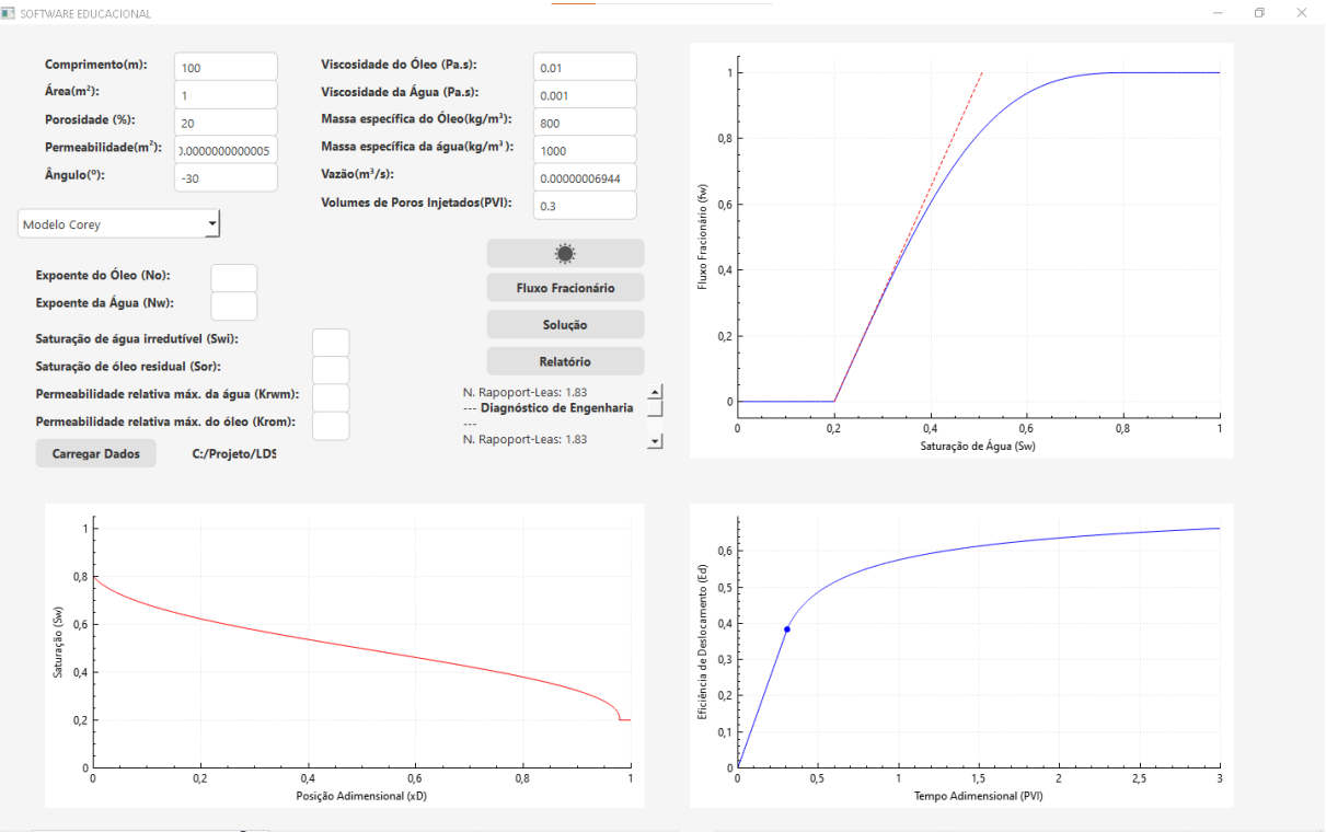
Figura 8.26: Tela do programa exibindo o perfil de saturação acelerado para injeção descendente em declive ( \alpha = -30^\circ )
