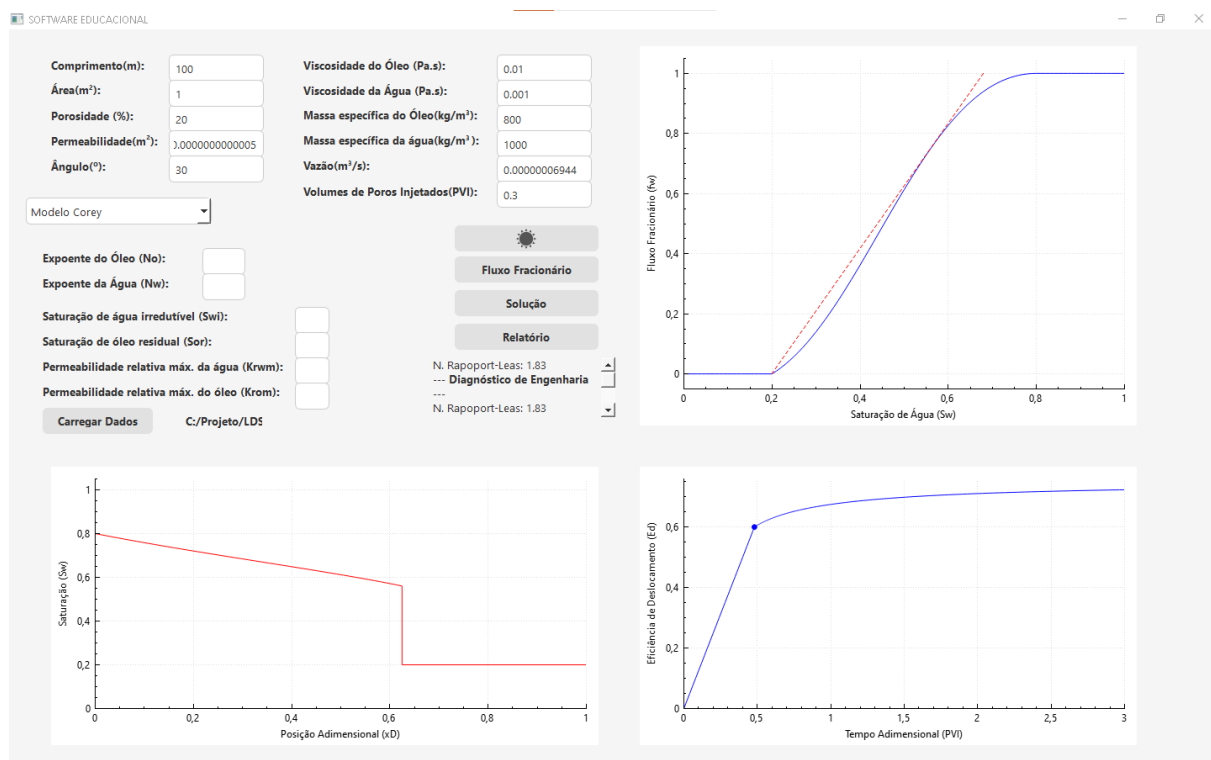
Figura 8.23: Tela do programa exibindo o perfil de saturação retardado para injeção ascendente em aclave ( \alpha = 30^\circ )
