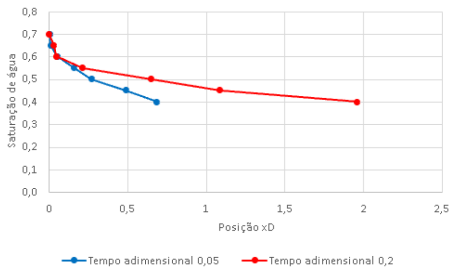
Figura 8.18: Perfil espacial de saturação de água, ilustrando a frente de choque de baixa saturação e a extensa onda de rarefação para os instantes de injeção t_D = 0,05 PVI e t_D = 0,2 PVI, computado em planilha para o Teste 1 (Cenário C)
