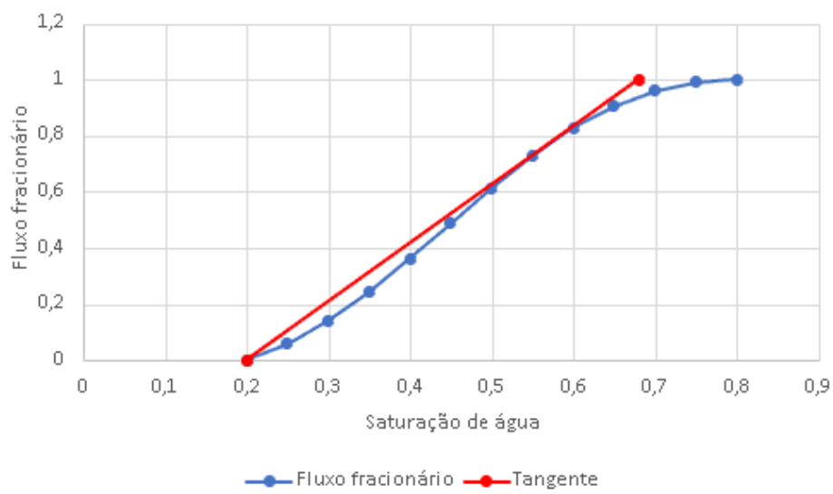
Figura 8.30: Gráfico analítico do fluxo fracionário sob influência gravitacional ( N_g = 1,13 ) e determinação discreta da secante de Welge (Teste 2, Cenário B)
