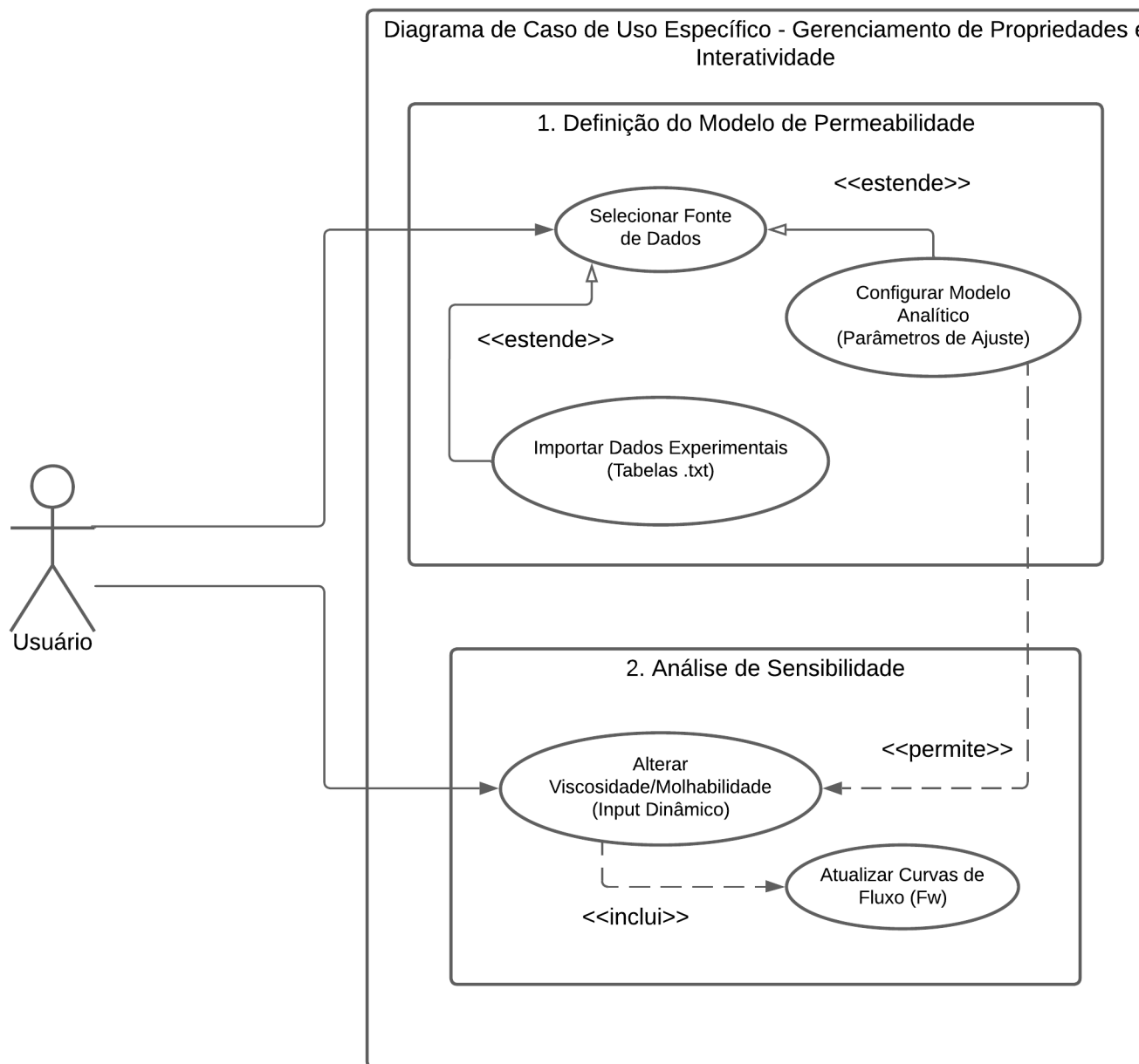
Figura 2.2: Diagrama de caso de uso específico – Gerenciamento de Propriedades e Interatividade
