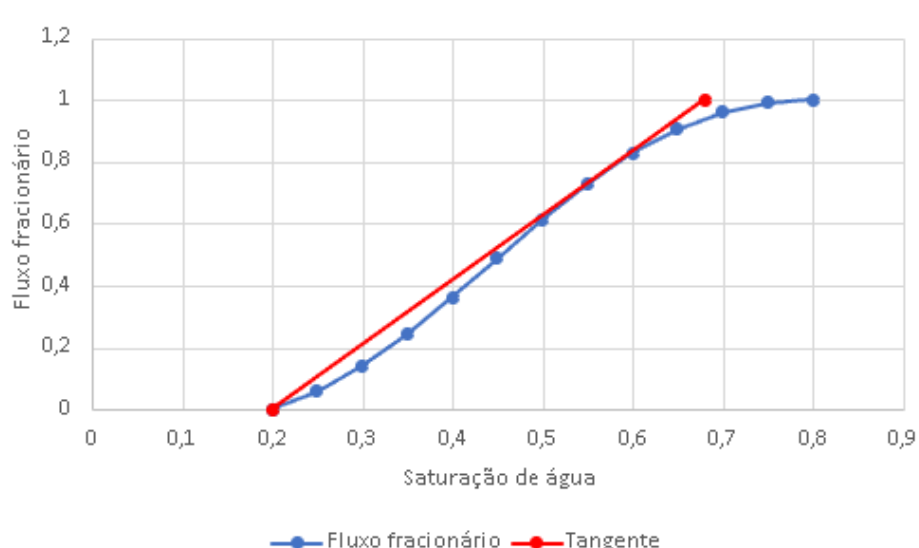
Figura 8.31: Gráfico analítico do fluxo fracionário sob influência gravitacional ( N_g = 1,13 ) e determinação discreta da condição de choque (Teste 2, Cenário B)
