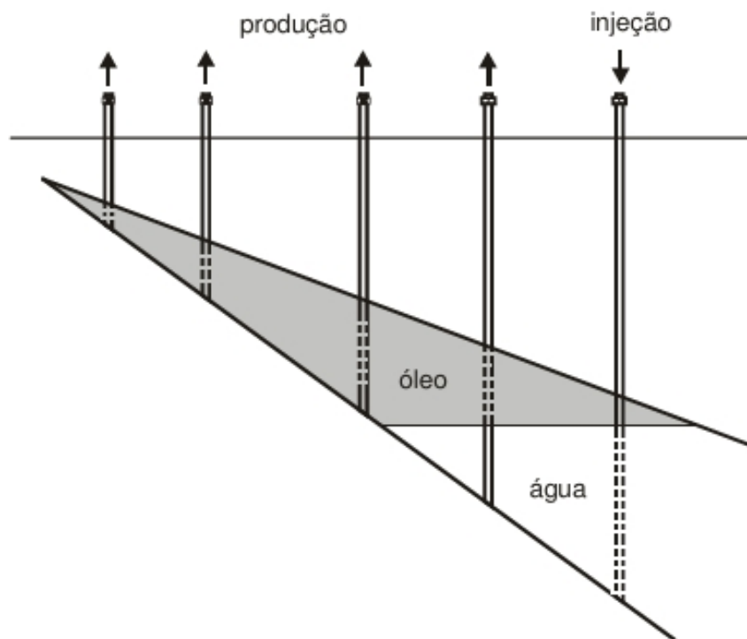
Figura 8.34: Injeção na base Retirada do livro (ROSA; CARVALHO; XAVIER, 2006)
