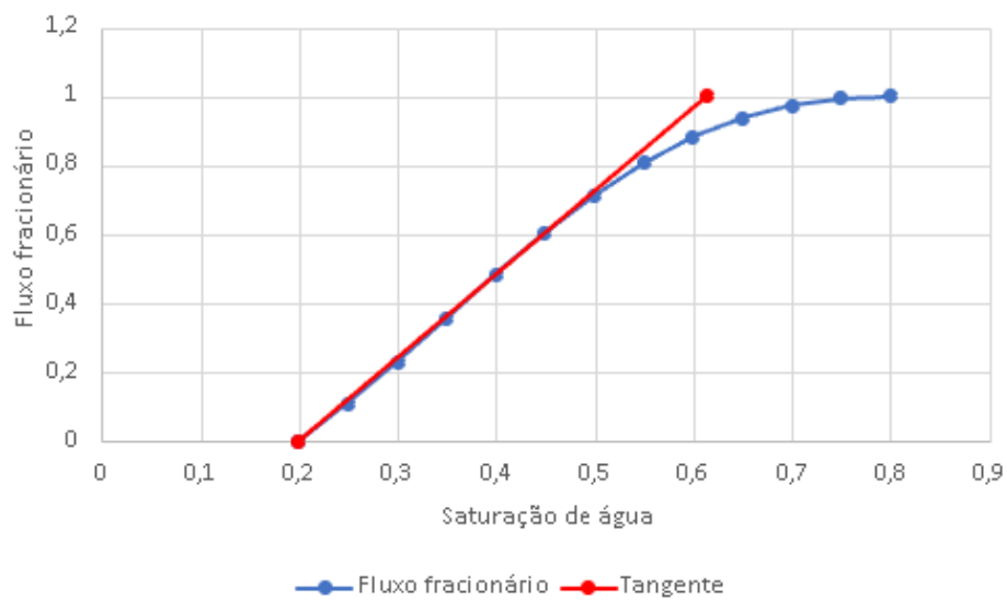
Figura 8.24: Gráfico analítico do fluxo fracionário e da condição de choque computados em planilha discreta para o modelo de Corey (Teste 2, Cenário A)
