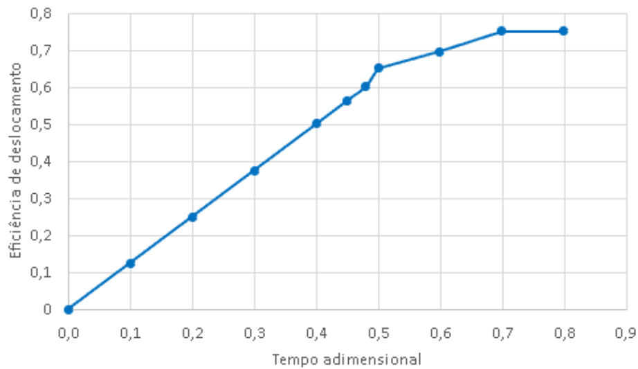
Figura 8.33: Histórico da evolução da eficiência de deslocamento volumétrico no escoamento ascendente (Teste 2, Cenário B)
