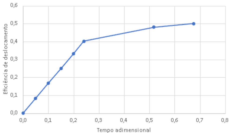
Figura 8.13: Histórico da eficiência de deslocamento em função do tempo adimensional para o Teste 1 (Cenário B)
