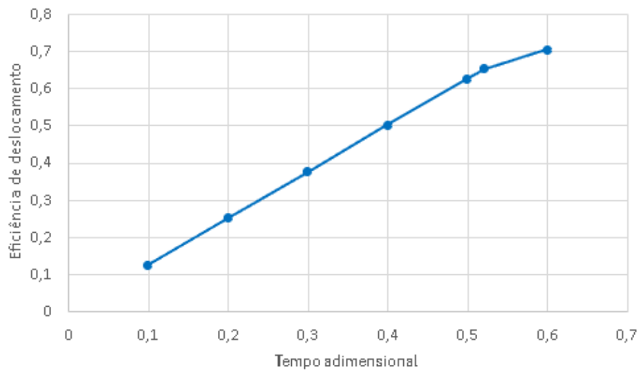
Figura 8.46: Histórico da eficiência de deslocamento volumétrico, refletindo o atraso cinemático imposto pelos parâmetros da rocha no modelo LET (Teste 3)
