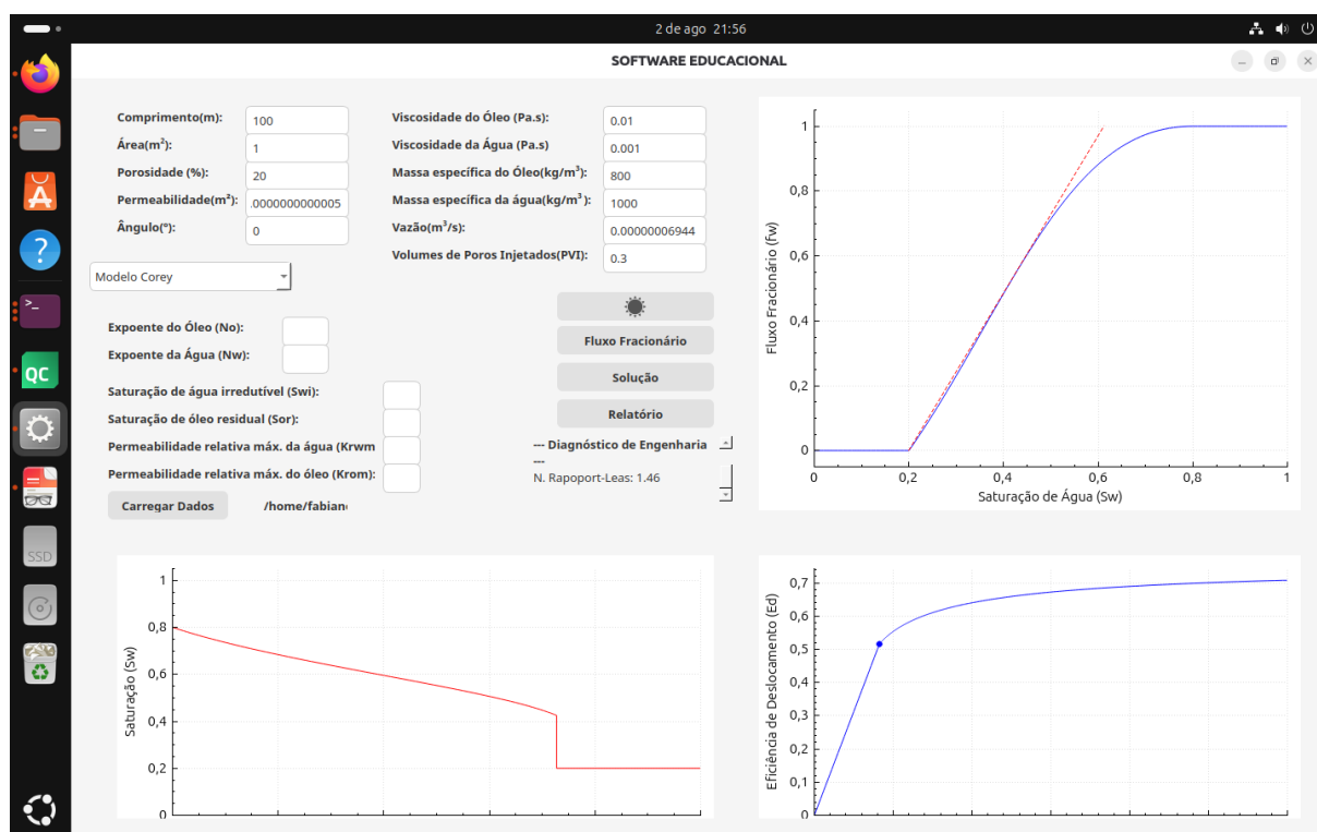
Figura 8.53: Interface gráfica do simulador em execução no sistema operacional Linux (Ubuntu), replicando os resultados analíticos do Cenário A do Teste 2
