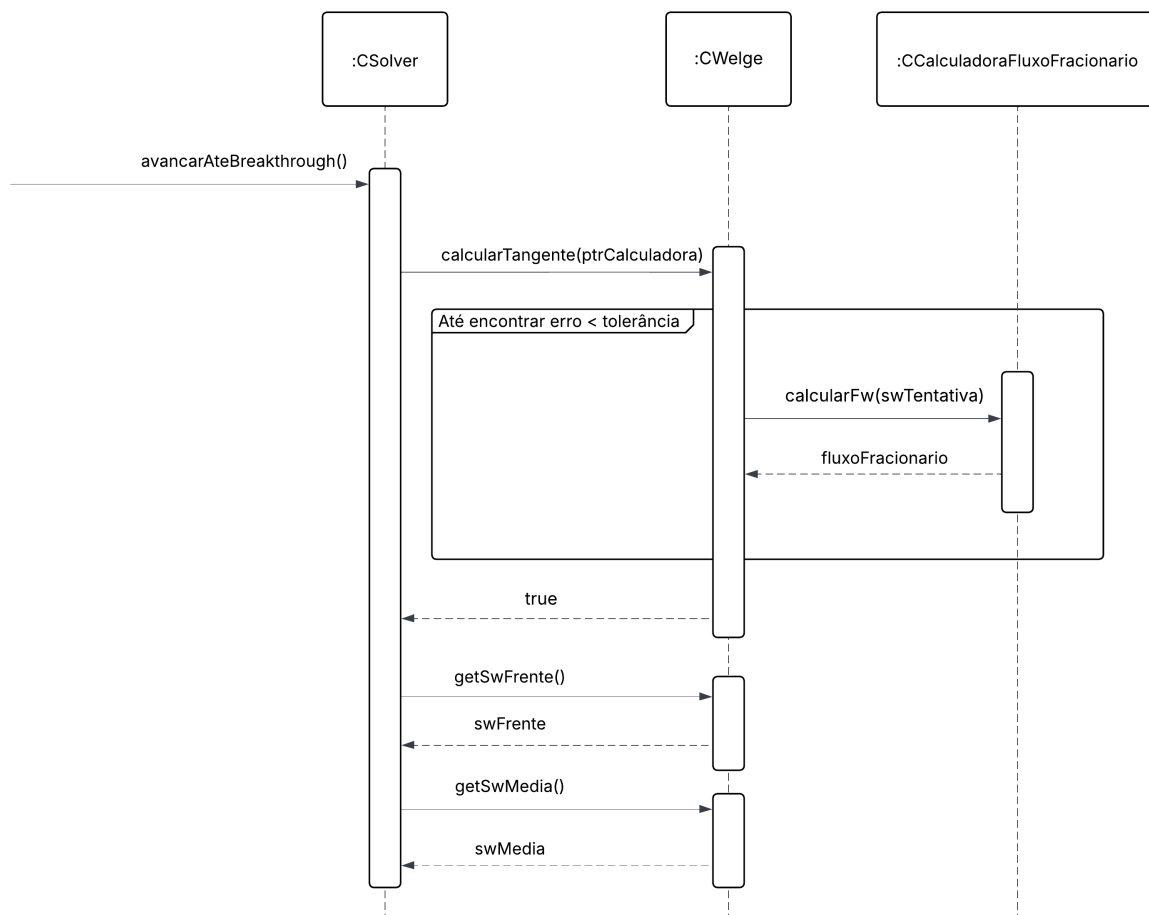
Figura 4.4: Diagrama de Sequência: Cálculo da Condição de choque
