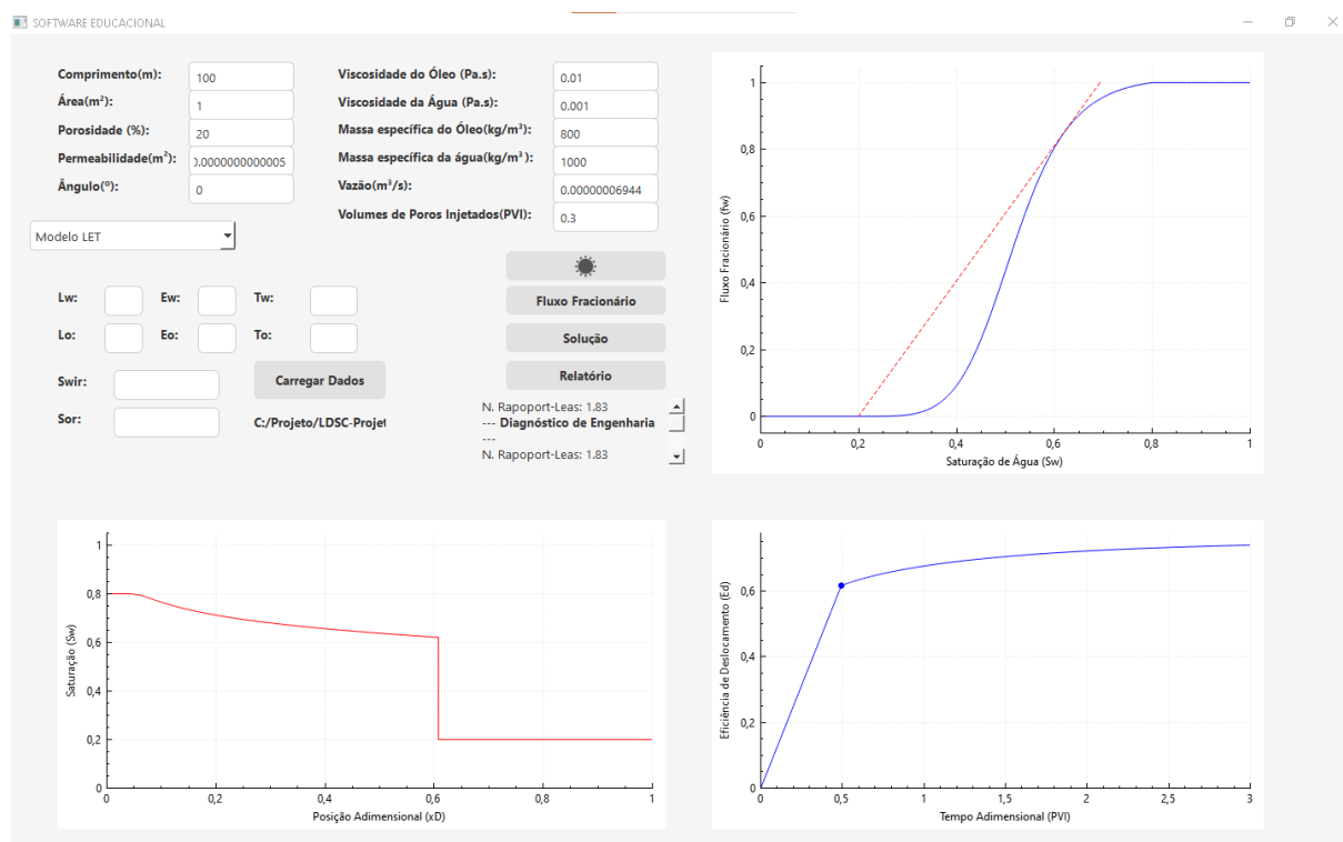
Figura 8.43: Painel principal do simulador processando o escoamento governado pelas curvas de permeabilidade do modelo LET
