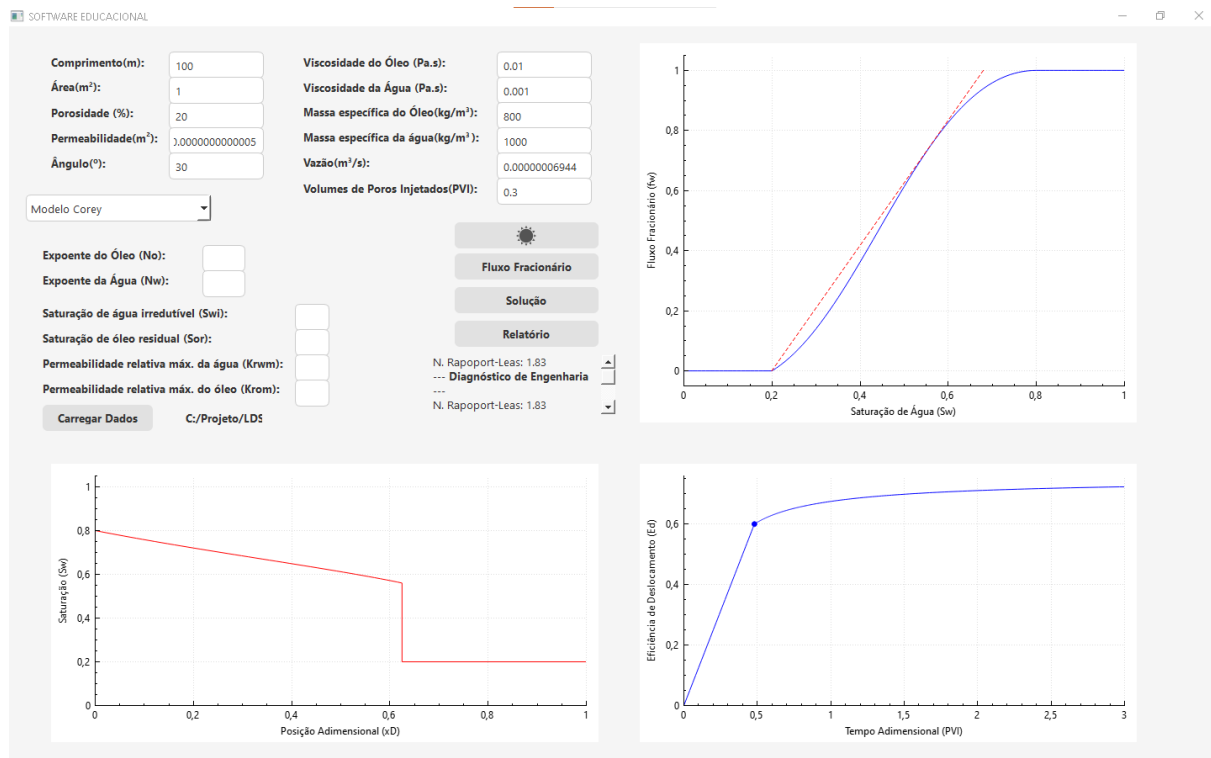
Figura 8.30: Tela do programa exibindo o perfil de saturação retardado para injeção ascendente em aclave ( \alpha = 30^\circ )
