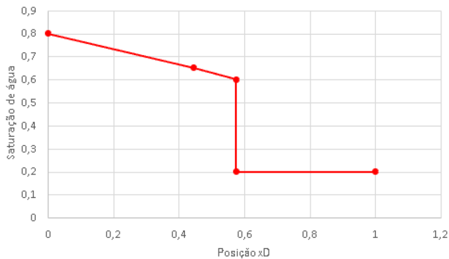
Figura 8.45: Perfil de saturação da água no instante t_D = 0,30 PVI, demonstrando a estabilidade da frente de choque verticalizada sob o equacionamento racional empírico (Teste 3)
