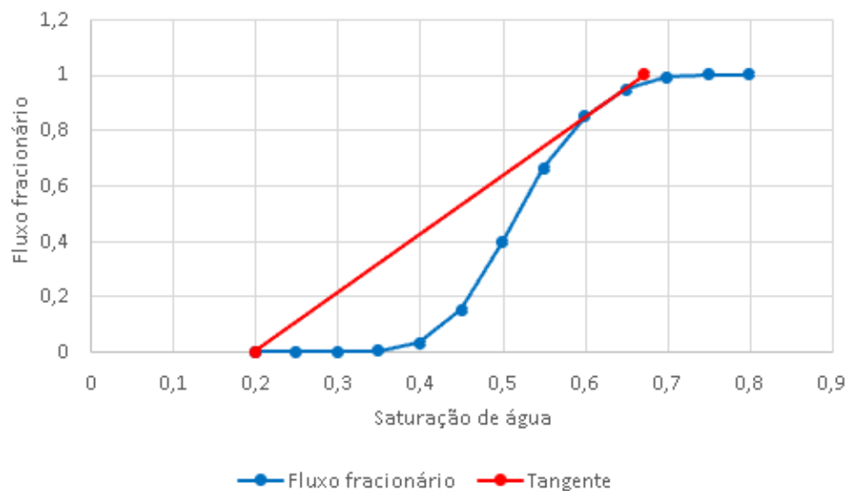
Figura 8.50: Gráfico do fluxo fracionário gerado pelo modelo de Chierici e a extrapolação da condição de choque até f_w = 1 para obtenção da saturação média (Teste 4)
