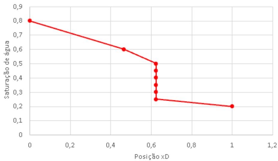
Figura 8.32: Perfil de propagação da saturação de água no instante t_D = 0,30 PVI, ilustrando o retardo do choque gravitacional (Teste 2, Cenário B)
