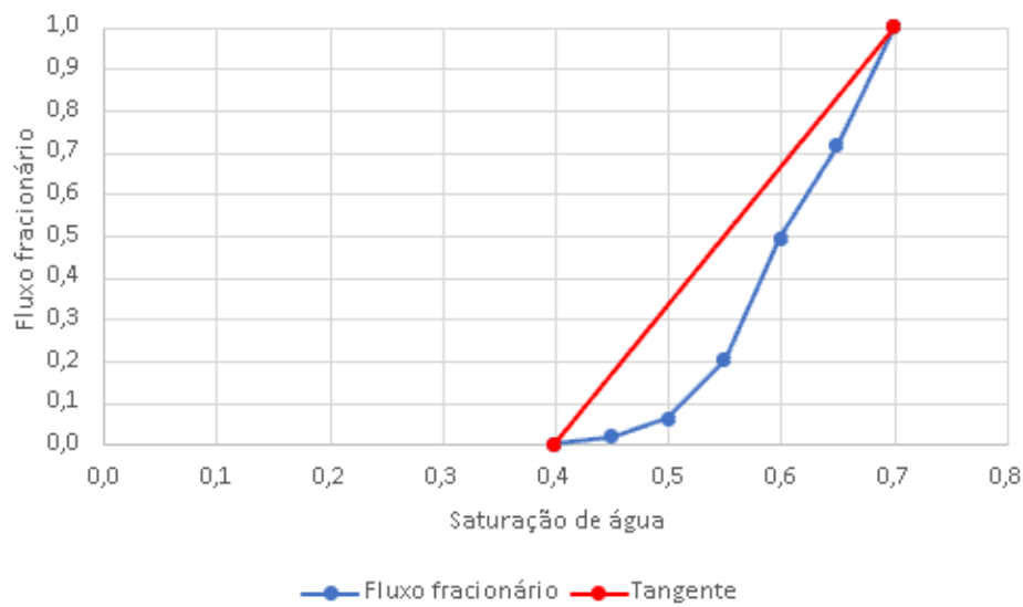
Figura 8.5: Gráfico analítico do fluxo fracionário e da condição de choque computados em planilha eletrônica para o Teste 1 (Cenário A)
