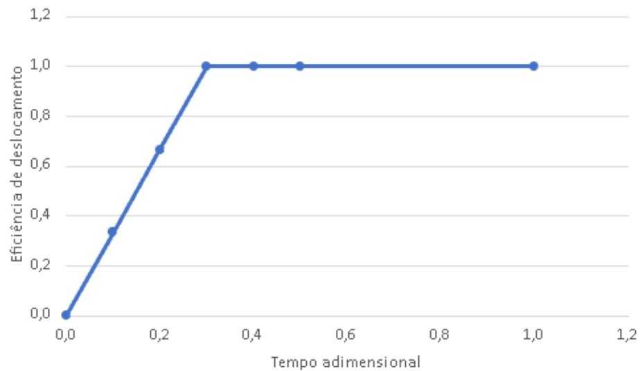
Figura 8.7: Histórico da eficiência de deslocamento em função do tempo adimensional para o Teste 1 (Cenário A)
