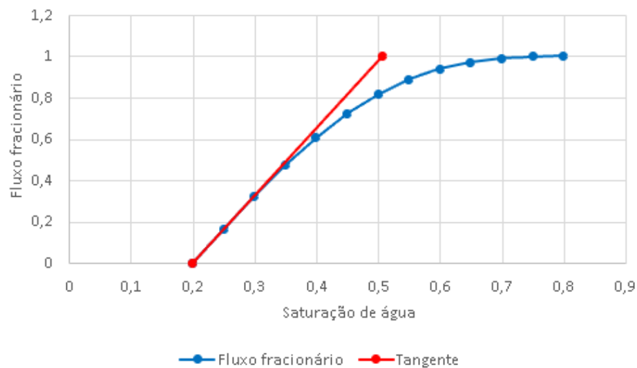
Figura 8.38: Gráfico analítico do fluxo fracionário em escoamento descendente e a aproximação discreta da condição de choque (Teste 2, Cenário C)
