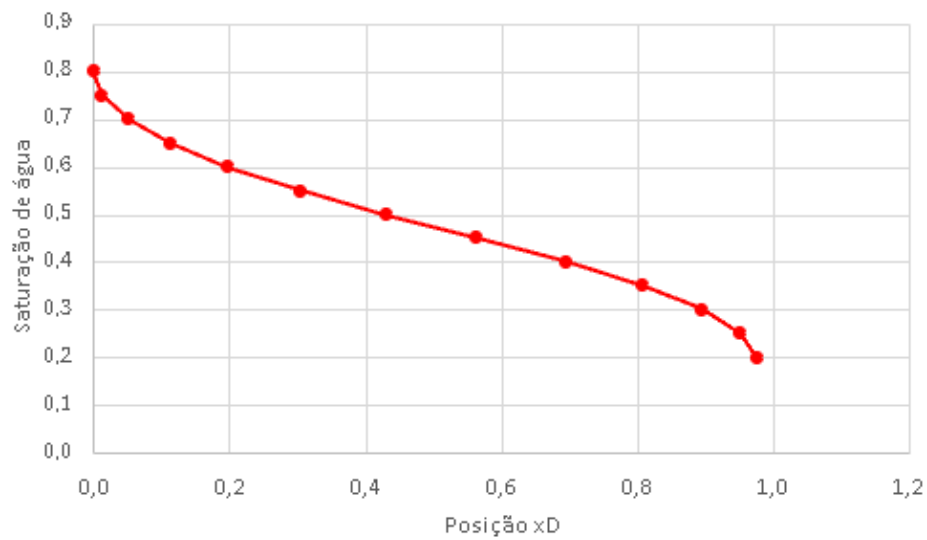
Figura 8.39: Perfil de propagação da saturação de água no instante t_D = 0,30 PVI, ilustrando a severa aceleração e o estiramento da onda de choque (Teste 2, Cenário C)
