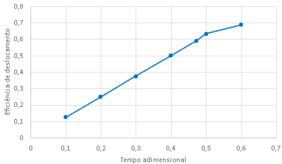
Figura 8.52: Histórico analítico da eficiência de deslocamento volumétrico associado ao escoamento regido pelas funções exponenciais de Chierici (Teste 4)
