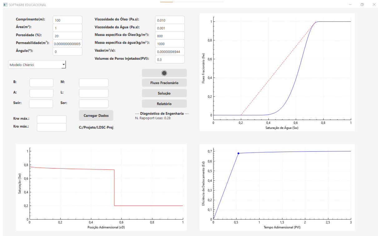
Figura 8.49: Painel de resultados da interface gráfica demonstrando a estabilidade computacional na interpolação do modelo de Chierici
