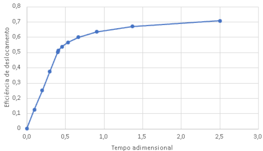
Figura 8.26: Histórico da evolução da eficiência de deslocamento ao longo do tempo adimensional (Teste 2, Cenário A)
