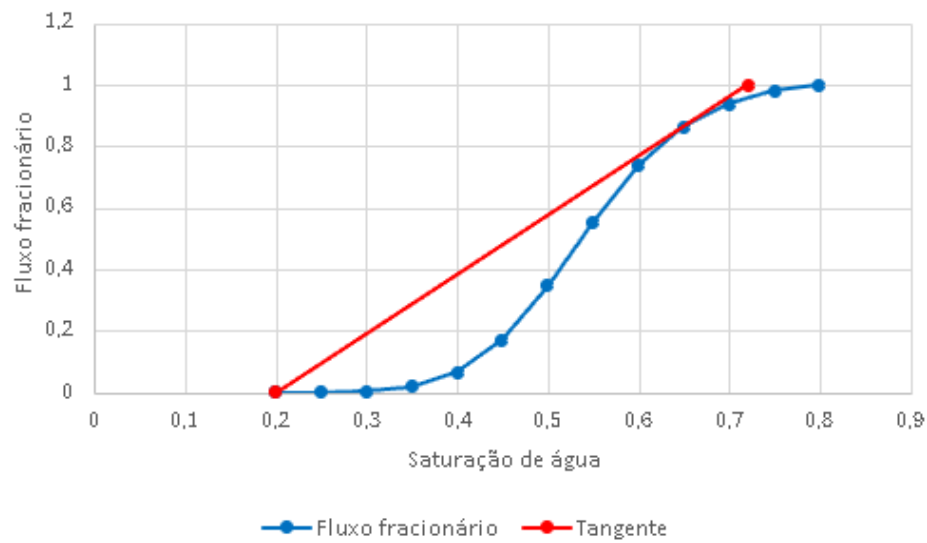
Figura 8.44: Gráfico do fluxo fracionário gerado a partir do modelo LET, evidenciando o extenso trecho convexo inicial e a determinação da condição de choque (Teste 3)
