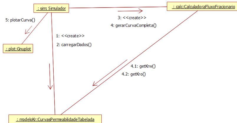
Figura 3.4: Diagrama de comunicação.
