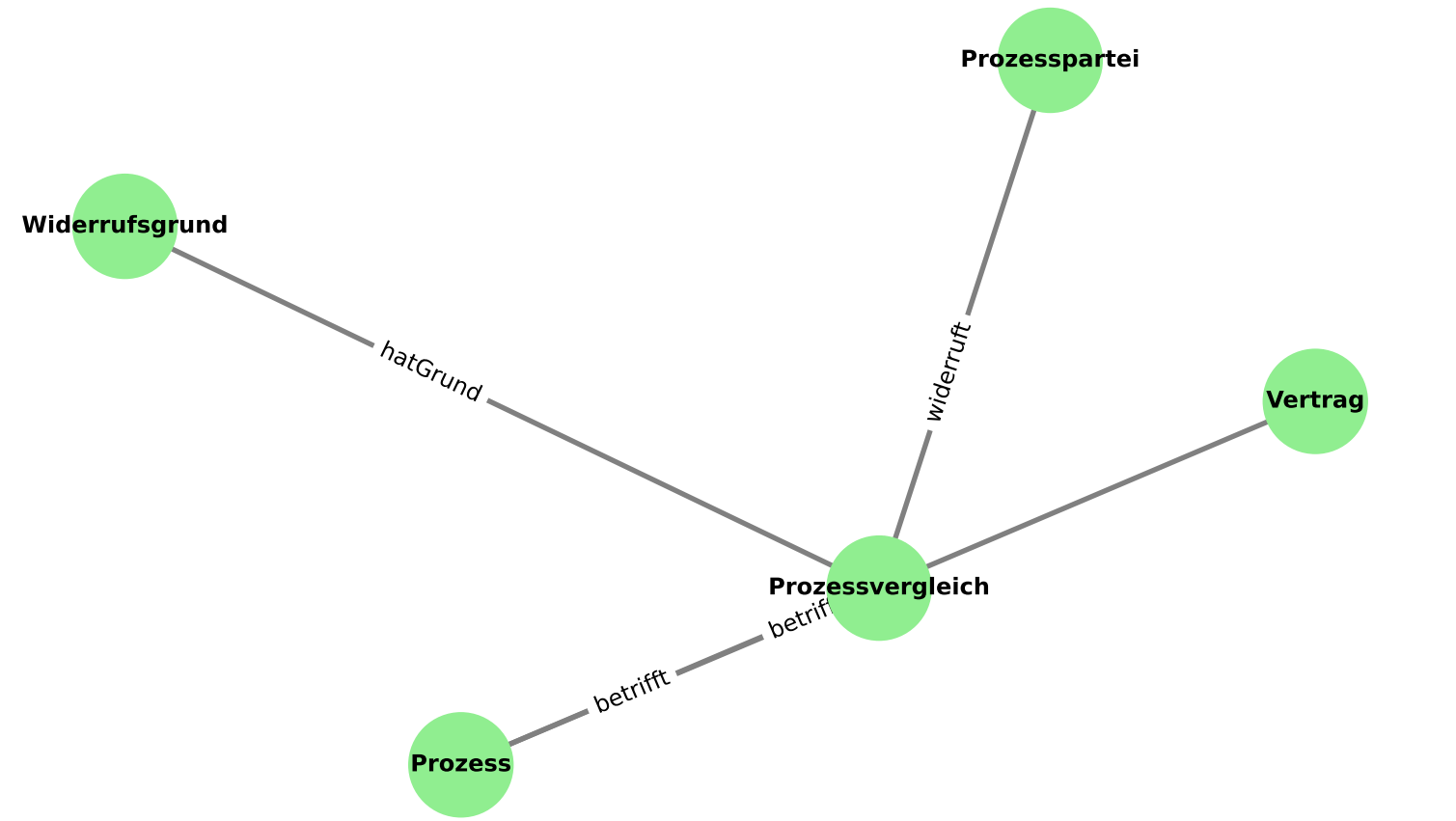
Cluster 104 - Generalisier
