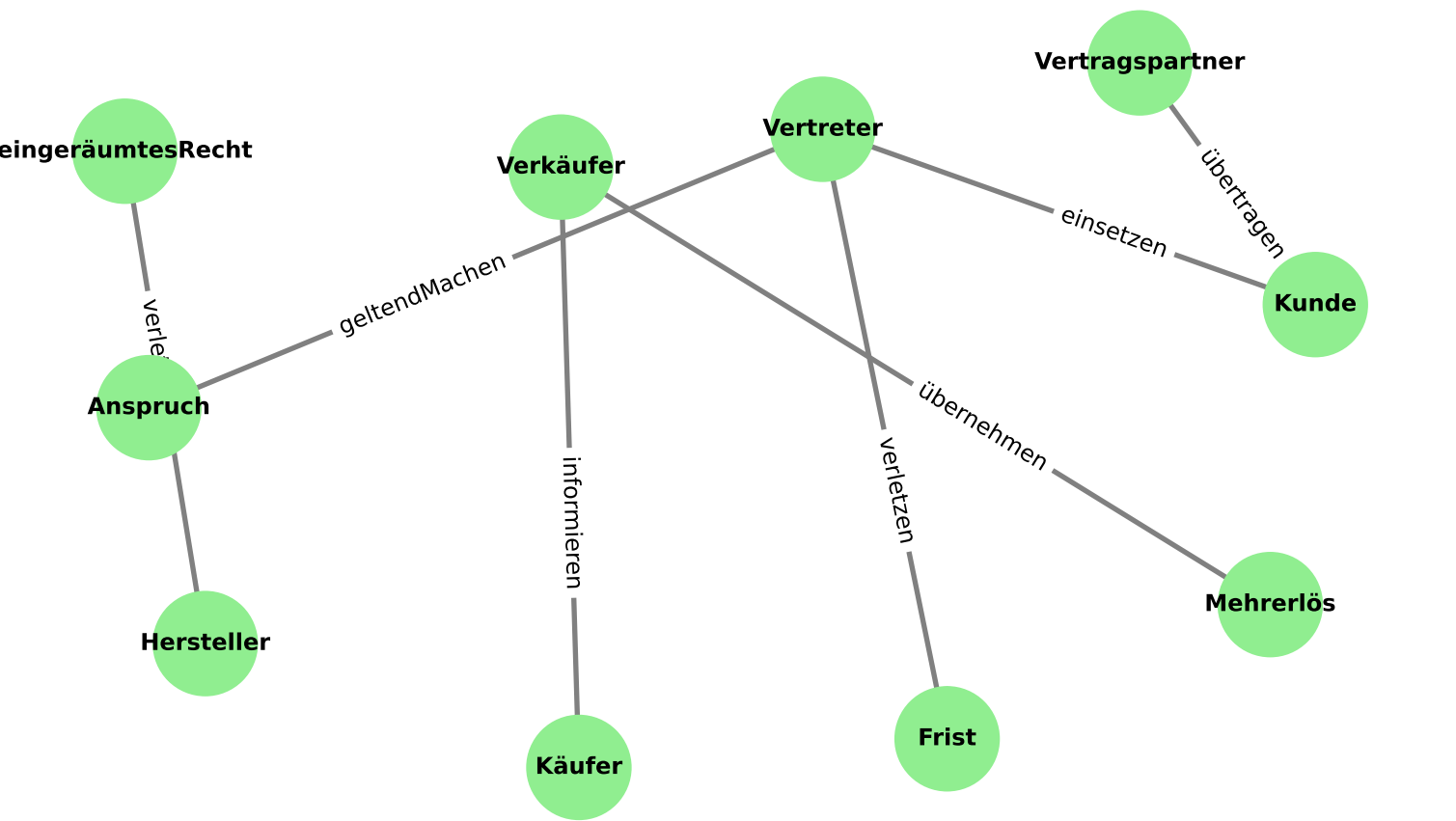
Cluster 102 - Generalisierung
