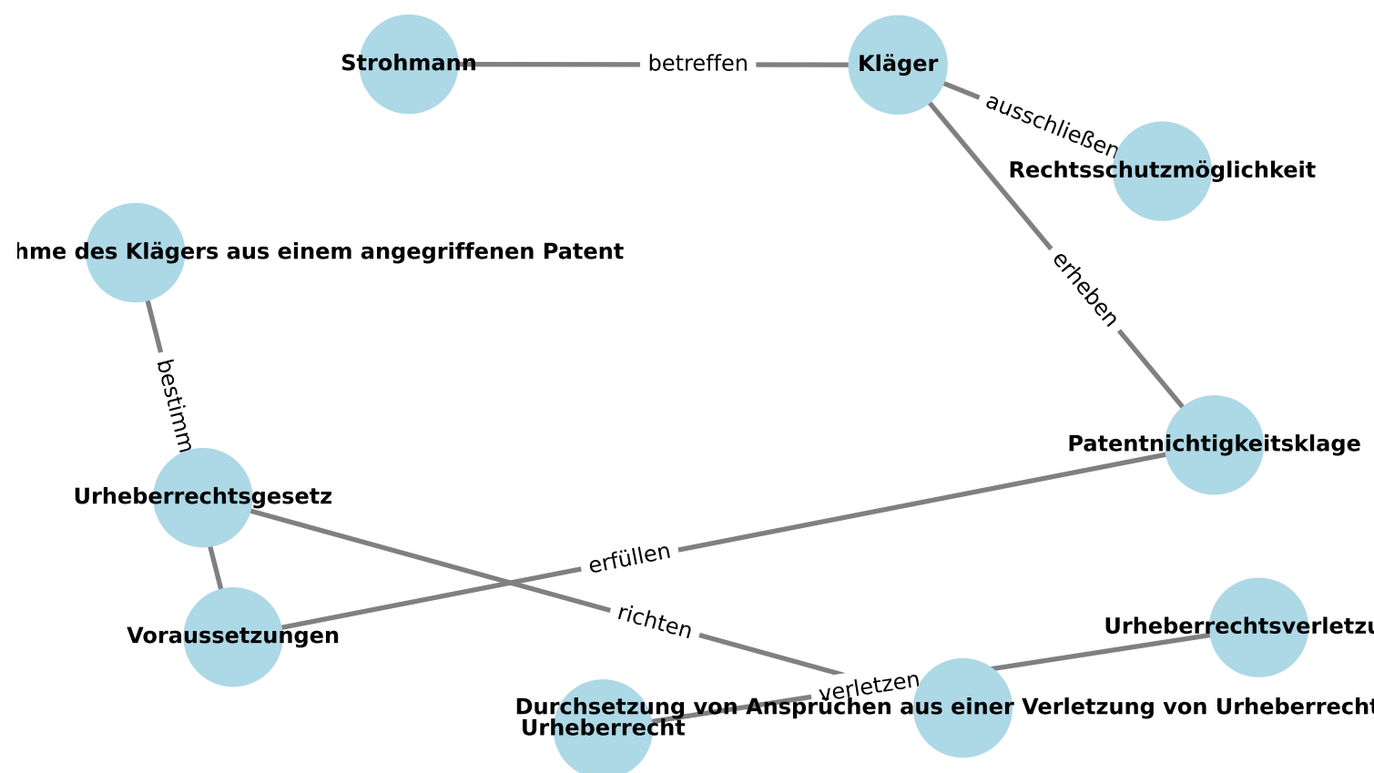
Cluster 10 - Détaillier
