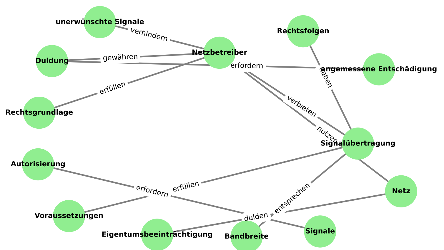
Cluster 1 – Generalisiert
