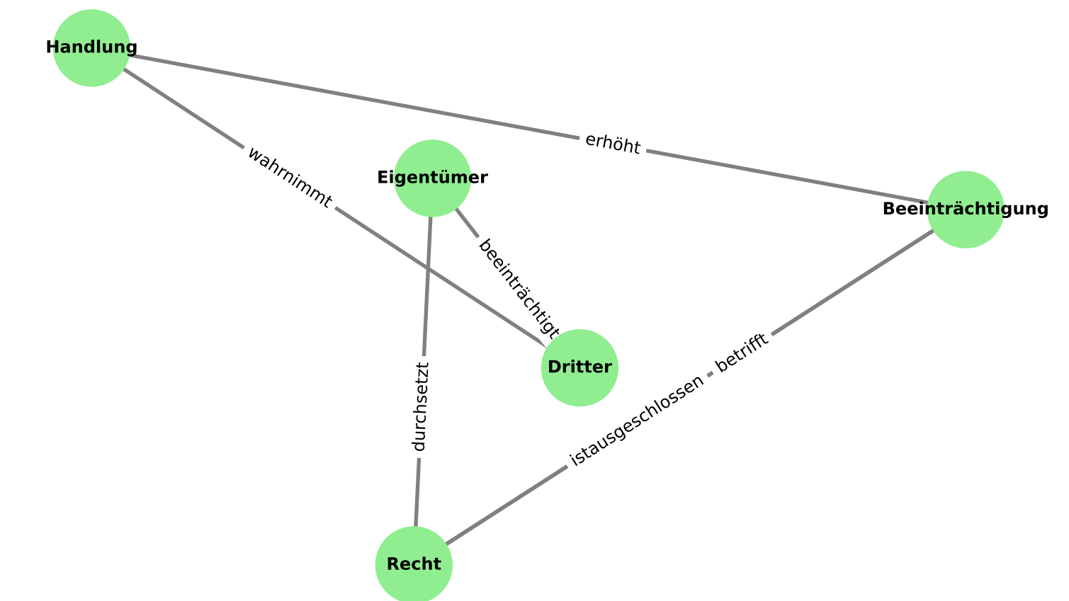
Cluster 100 – Generalisierung
