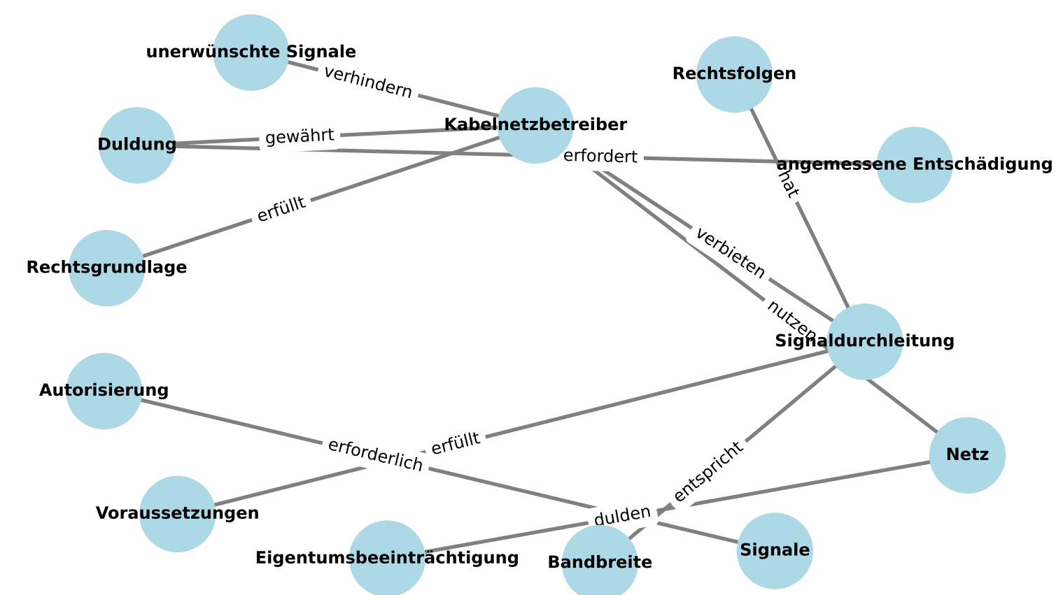
Cluster 1 - Detailliert
