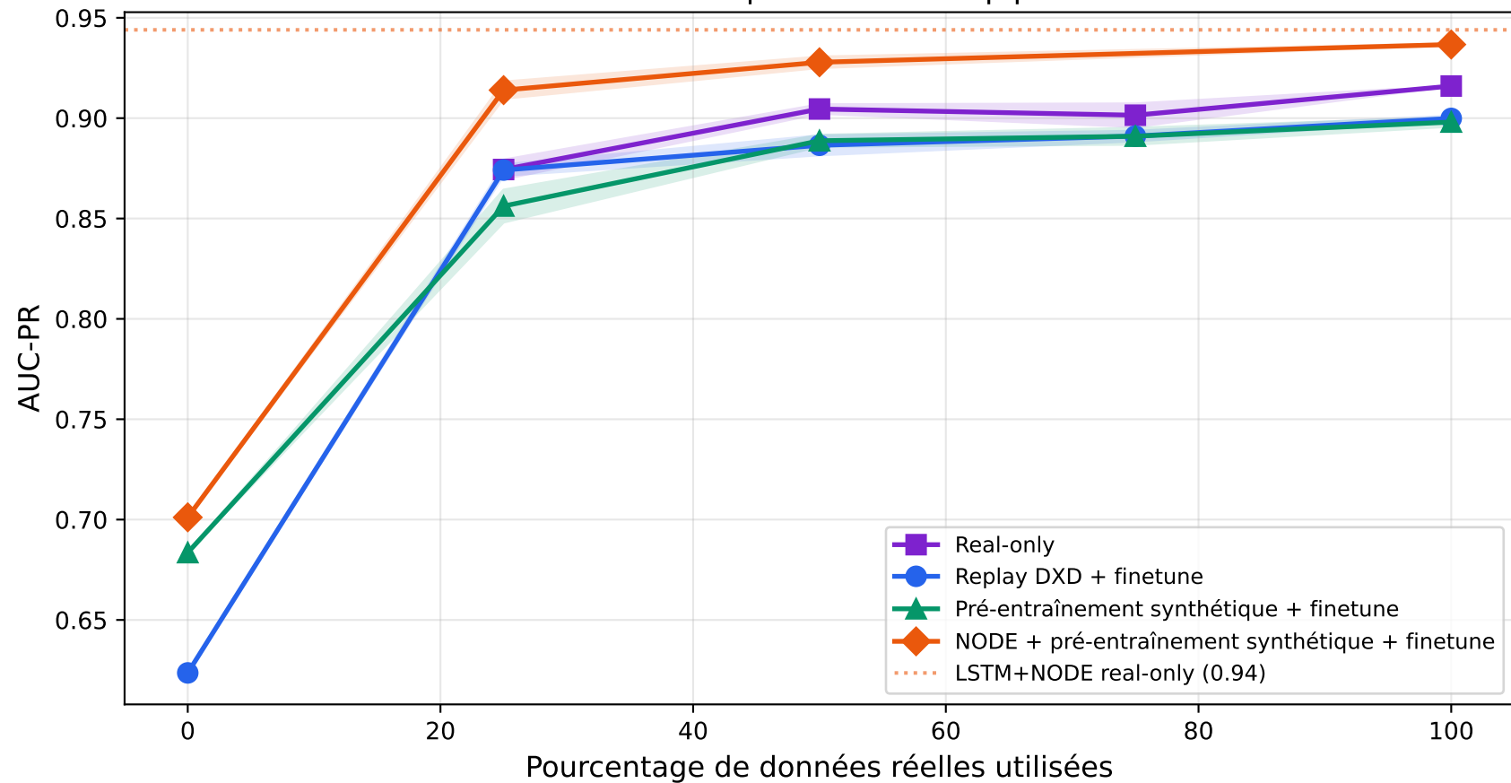
D4 h2s — Comparaison des 4 pipelines
