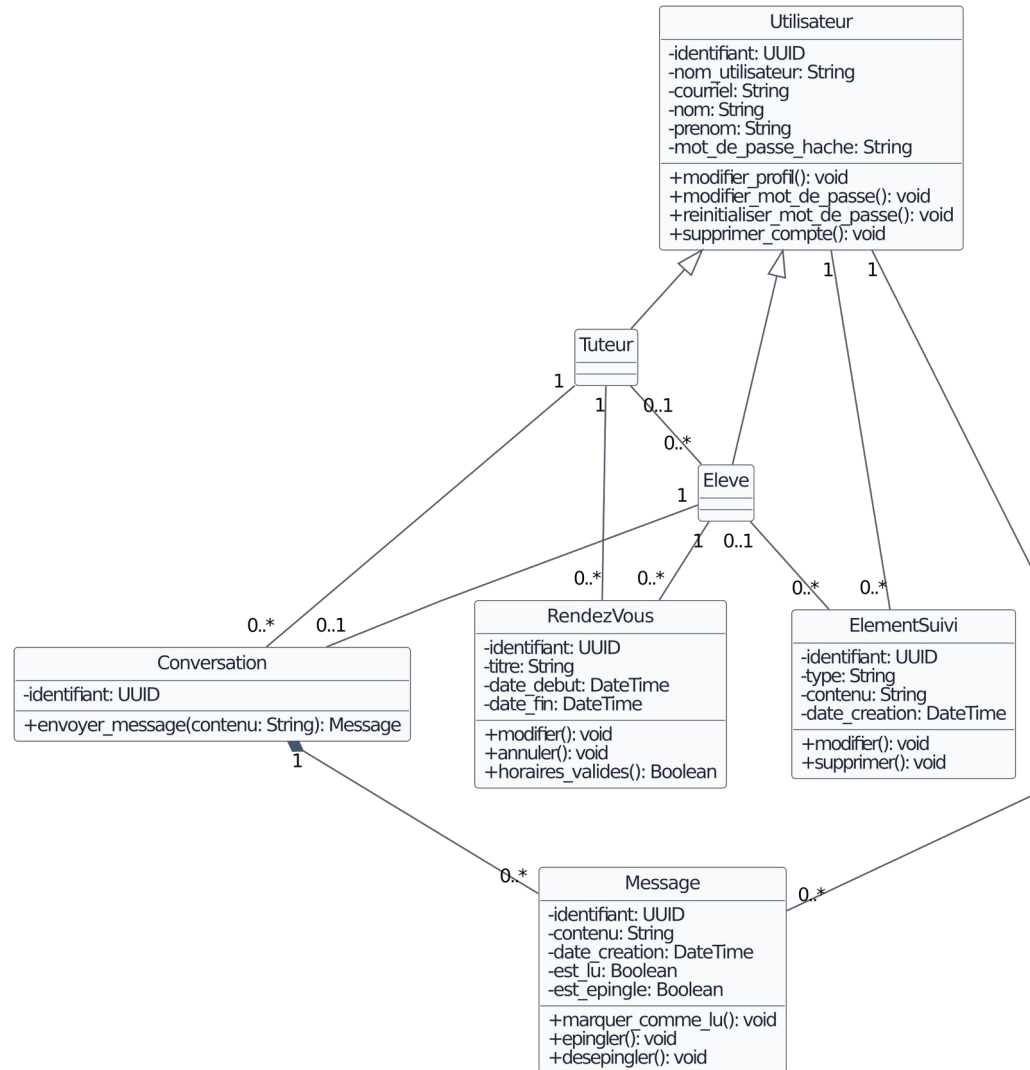
Figure A.1 — Diagramme de classes métier HomeSkolar — version simplifiée validée
