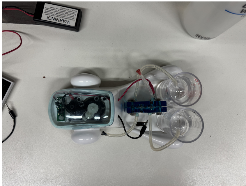
Abbildung 5: Hydrocar zusammengebaut
