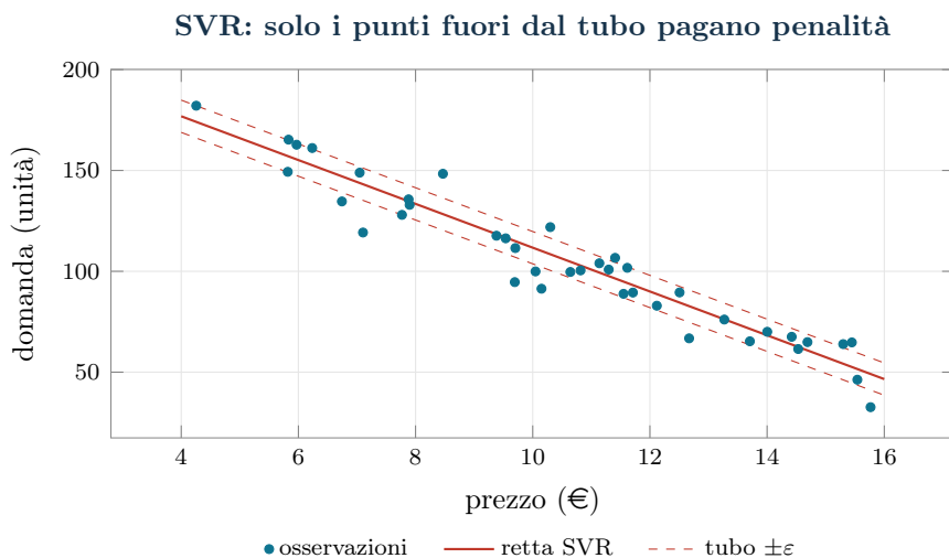
Figura 15.3: Support Vector Regression sulla relazione prezzo–domanda: le 40 osservazioni, la retta stimata e il tubo di tolleranza \pm\varepsilon = 8 : solo i 14 punti fuori dal tubo pagano penalità e determinano la retta.
