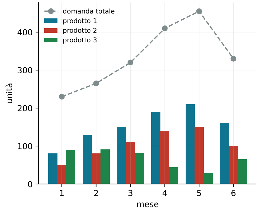
Piano di produzione ottimo (LP)
