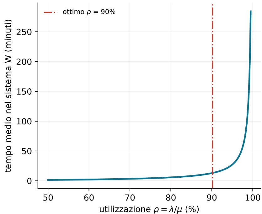
Il muro dell'utilizzazione: W esplode per \rho \rightarrow 1
