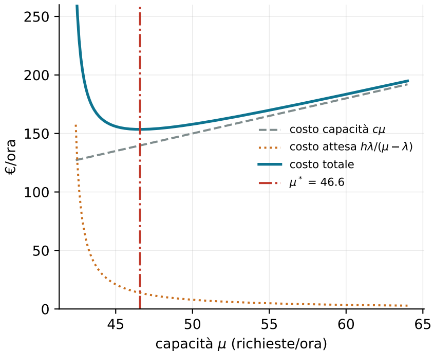
Il costo totale è convesso in \mu
