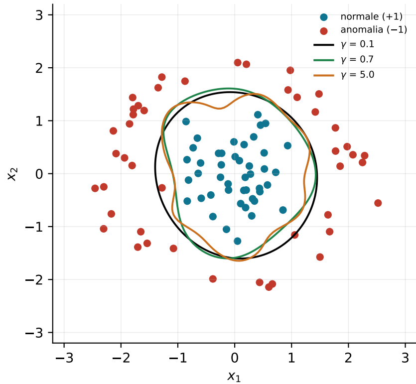
Kernel RBF: frontiere non lineari da un QP convesso
