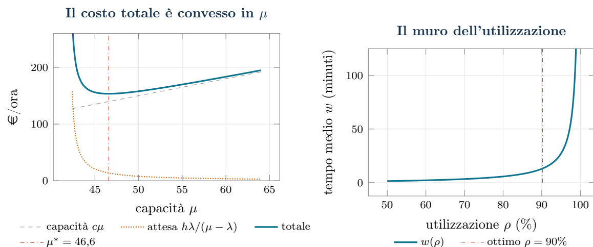
Figura 11.1: A sinistra: le due componenti del costo (capacità, crescente; attesa, decrescente) e il costo totale, convesso, con il minimo in \mu^* = 46,6 . A destra: il “muro dell'utilizzazione” — il tempo medio nel sistema w in funzione dell'utilizzazione \rho : oltre il 90% l'attesa esplode in modo iperbolico.
