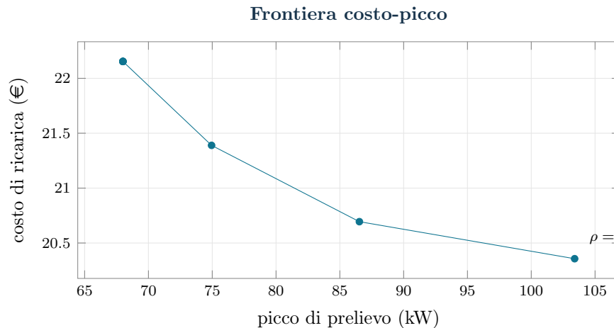
Figura 10.2: Frontiera costo-picco ottenuta variando il peso \rho del picco nell'obiettivo: ogni punto è una strategia di ricarica ottima. Ridurre il picco da 103 a 75 kW costa circa un euro a notte; il punto \rho \geq 0,2 raggiunge il picco minimo possibile (68 kW) al costo più basso che lo consente.
