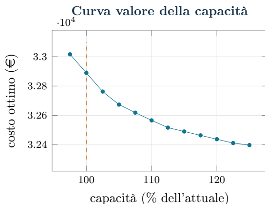
Figura 4.3: Costo totale ottimo in funzione della capacità disponibile (in % dell'attuale; la linea tratteggiata arancione segna la capacità corrente): curva convessa e decrescente, interrotta a sinistra dove il problema diventa inammissibile.
