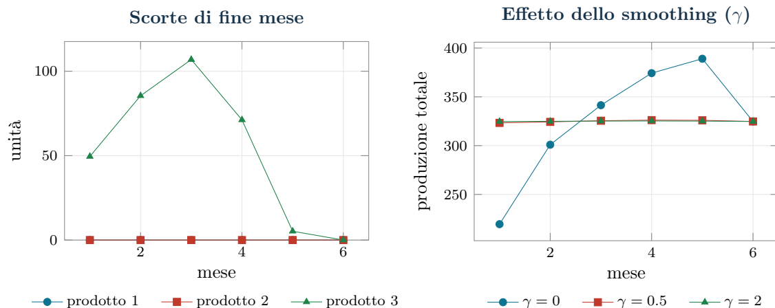
Figura 4.2: A sinistra: scorte di fine mese per prodotto — solo il prodotto 3 usa il magazzino (strategia di pre-build), e le scorte si azzerano nel mese finale. A destra: produzione totale mensile per tre valori del peso di smoothing \gamma : già con \gamma = 0,5 il profilo diventa quasi piatto.
