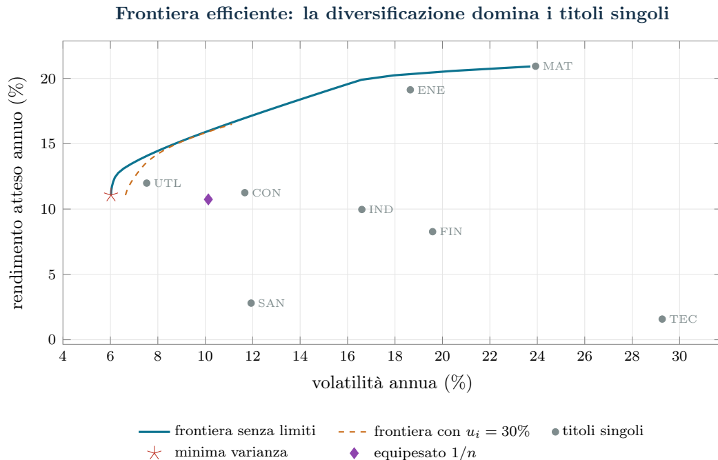
Figura 6.1: Piano rischio-rendimento: gli otto titoli (punti grigi), la frontiera efficiente senza limiti (linea teal), la frontiera con tetto del 30% per titolo (tratteggiata arancione), il portafoglio di minima varianza (stella rossa) e l'equipesato 1/n (rombo viola), che risulta dominato.
