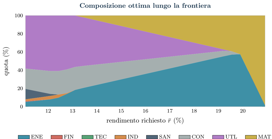
Figura 6.2: Composizione del portafoglio ottimo (aree impilate, in %) al crescere del rendimento richiesto \bar{r} : a sinistra domina il mix difensivo (UTL, CON, SAN), verso destra il portafoglio si concentra progressivamente sui titoli ad alto rendimento (MAT, ENE) fino al portafoglio monotitolo all'estremo.
