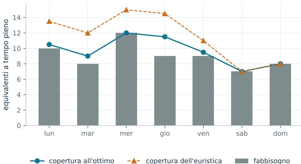
EX 13: costo 7060 contro euristica 8410
