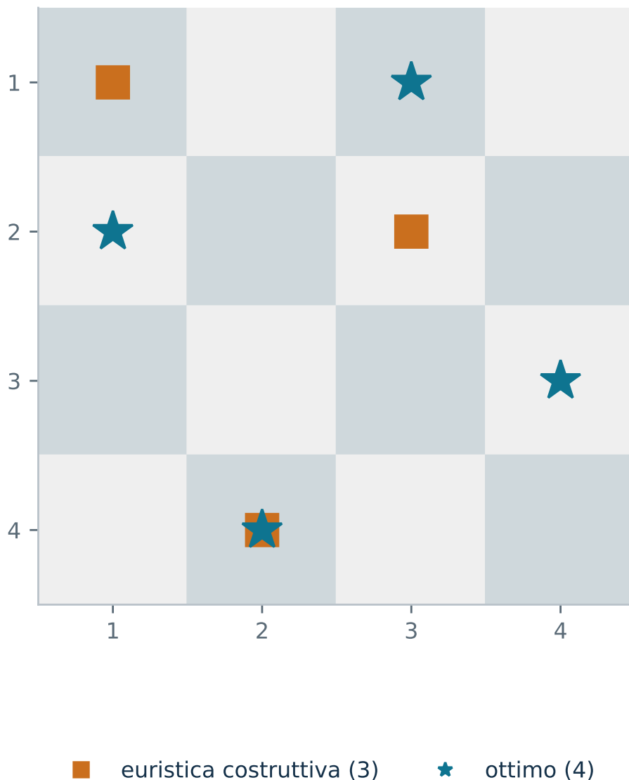
Figura 9: EX 9: le tre regine piazzate dall'euristica e le quattro della soluzione ottima.
