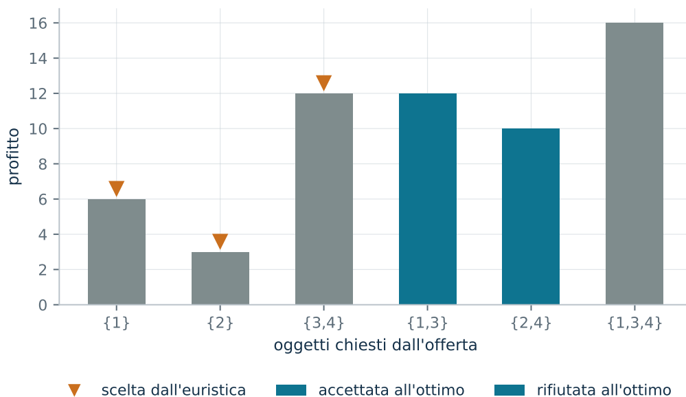
10.2: euristica 21 <= ottimo 22 <= duale 23
