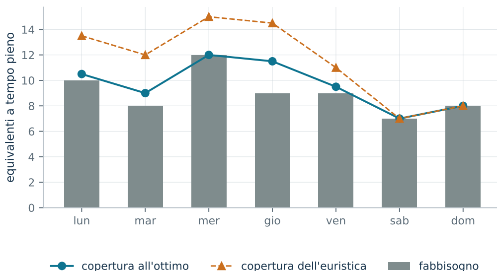
EX 14: costo 7060 contro euristica 8410
