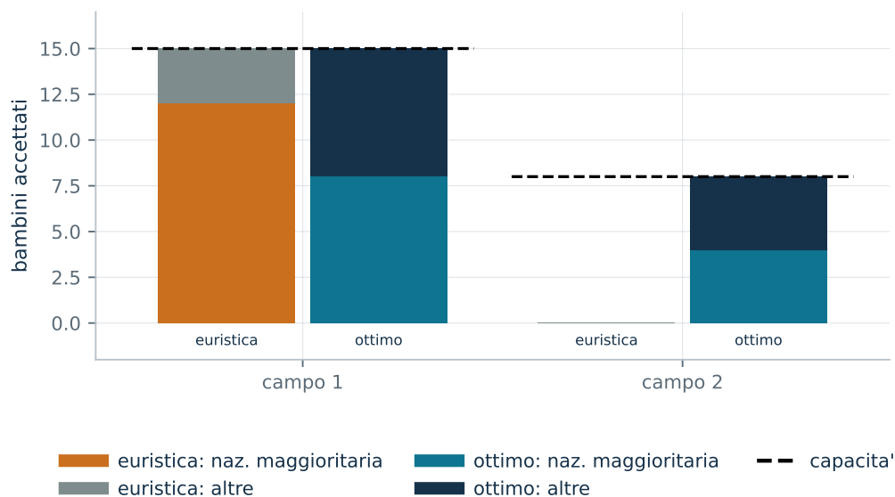
10.6: euristica 15 contro ottimo 23
