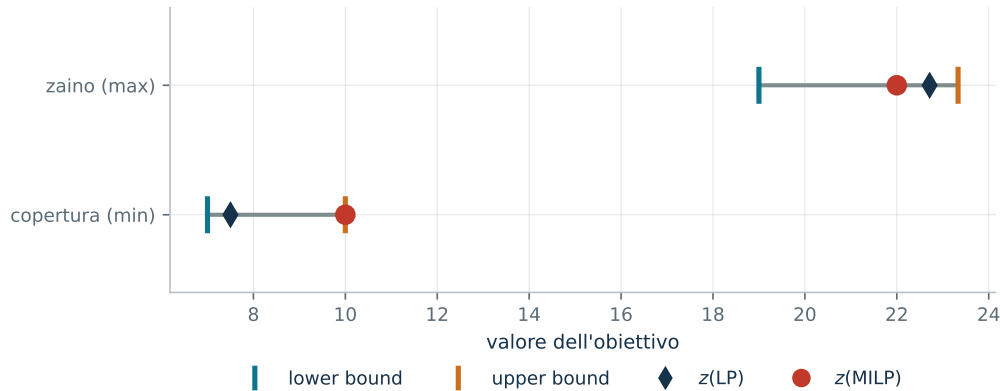
Figura 2.1: I due esempi. In un minimo il bound duale sta a sinistra dell'ottimo e l'euristica a destra; in un massimo i ruoli si scambiano.
