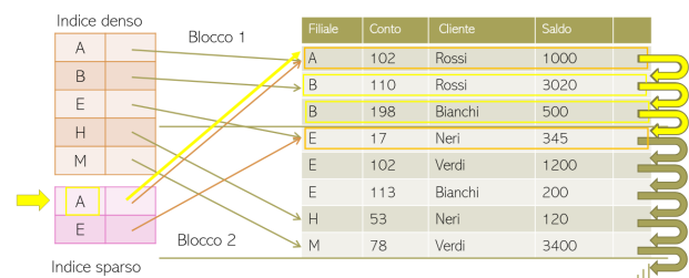
Figura 41: Esempio di ricerca con indice primario sparso
