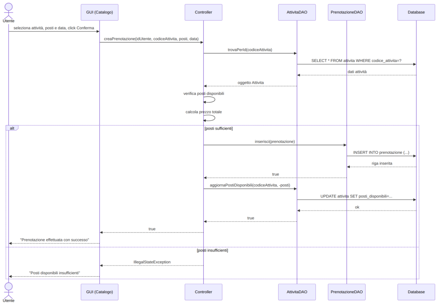
Figura 2 — Sequence diagram del flusso di creazione di una prenotazione
