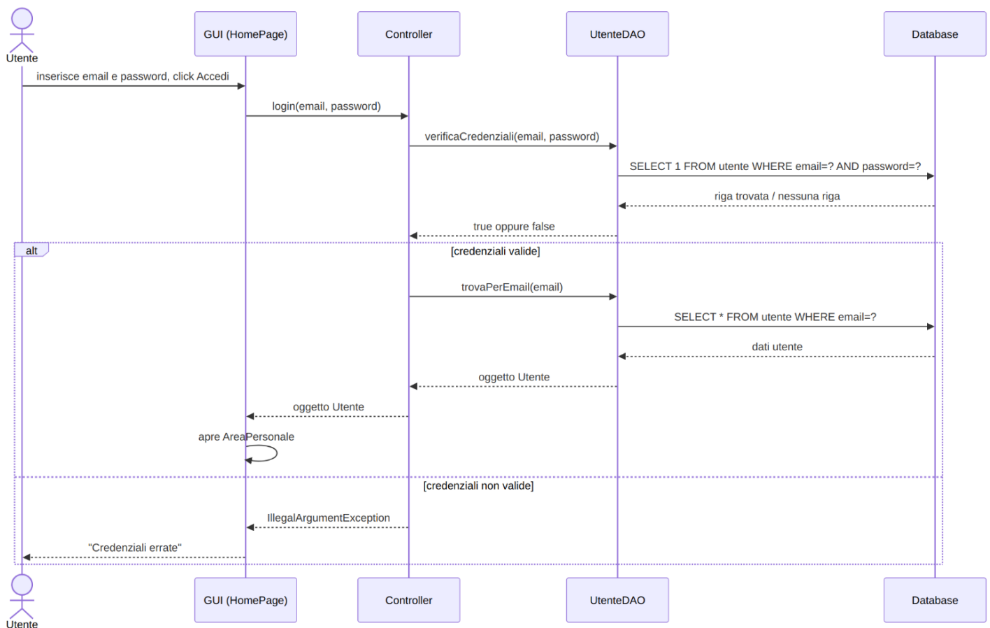
Figura 1 — Sequence diagram del flusso di login
