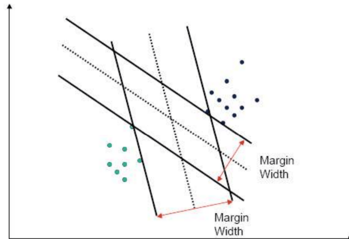
Figura 13.3: Iperpiani separatori diversi hanno margini diversi.
