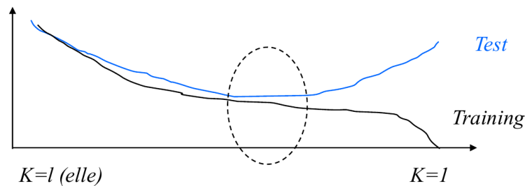
Figura 5.19: Comportamento del K-NN: da k = l (rigido) a k = 1 (flessibile) l'errore di training scende sempre, quello di test ha forma a U.
