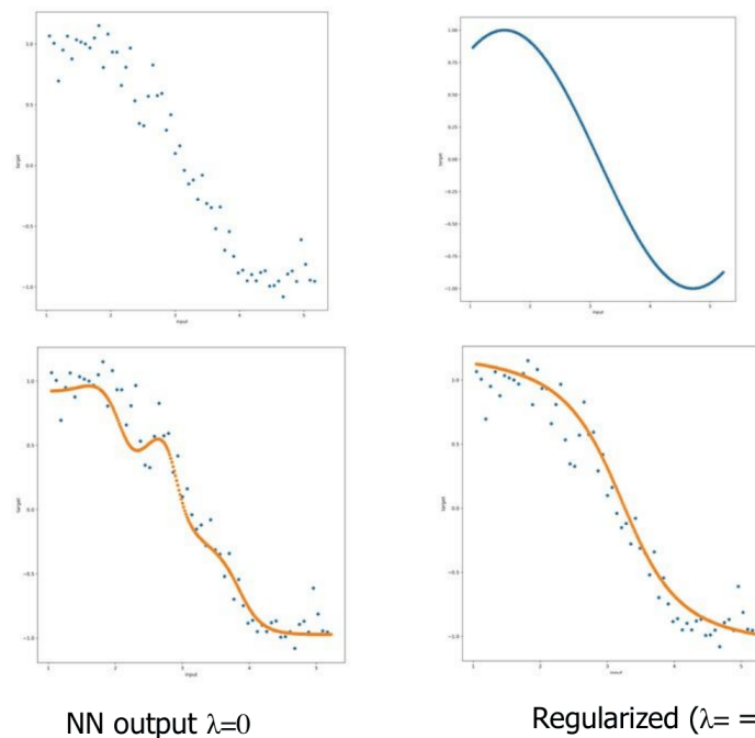
Figura 8.8: Regressione univariata: rete senza regolarizzazione ( \lambda = 0 ) e regolarizzata ( \lambda = 0,01 ).
