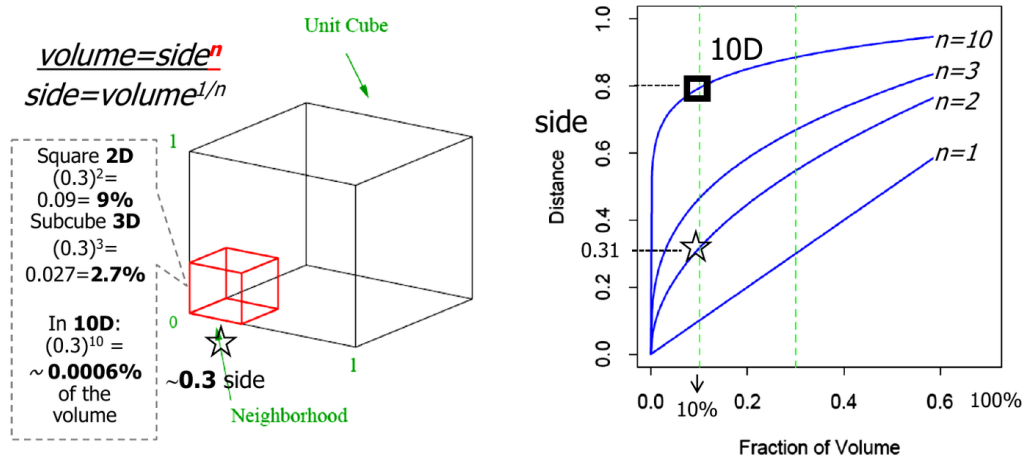
Figura 5.23: Maledizione della dimensionalità: lato del sottocubo necessario per catturare una frazione r del volume, al variare della dimensione n .
