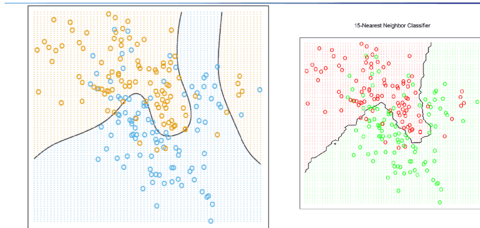
Figura 5.21: Confine di Bayes ottimo (sinistra) e confine del 15-NN (destra): il 15-NN è molto vicino all'ottimo, coerentemente con il minimo dell'errore di test nella figura precedente.
