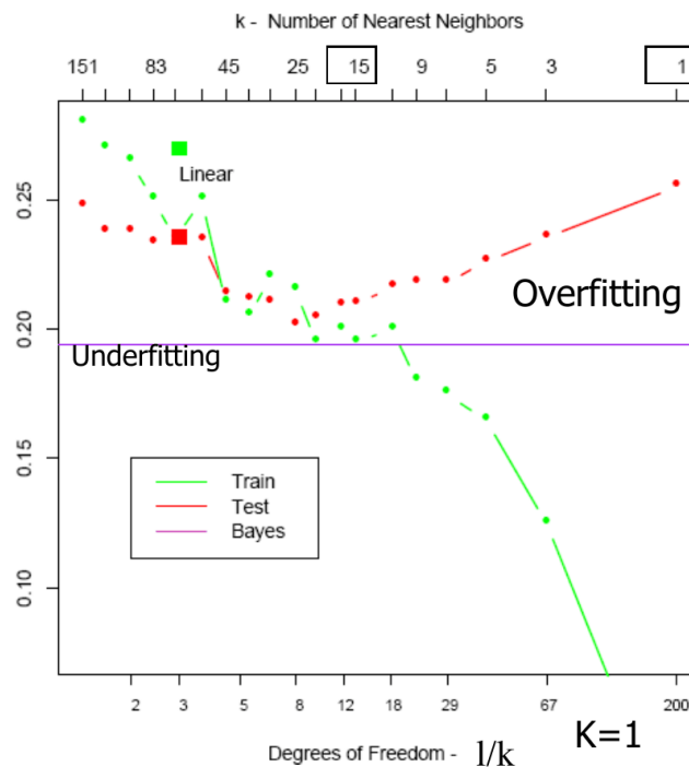
Figura 5.20: Curve di errore del K-NN al variare di k (training di 200 punti, test di 10000). I quadratini sono il modello lineare, la linea viola l'errore ottimo di Bayes.
