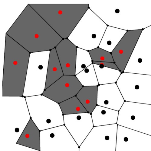
Figura 5.18: Diagramma di Voronoi: il confine del 1-NN segue i lati delle celle tra punti di classi diverse.
