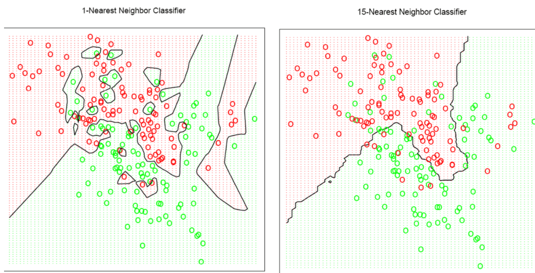
Figura 5.17: Confini di decisione del 1-NN (sinistra) e del 15-NN (destra) sullo stesso problema.
