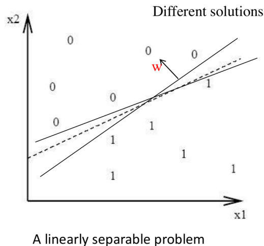
Figura 5.4: Un problema linearmente separabile ammette molti iperpiani separatori; \mathbf{w} è ortogonale all'iperpiano.
