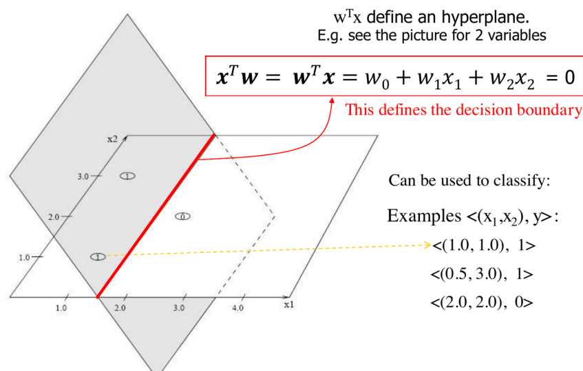
Figura 5.2: Iperpiano \mathbf{w}^T \mathbf{x} e la sua intersezione con il piano degli input: il confine di decisione.
