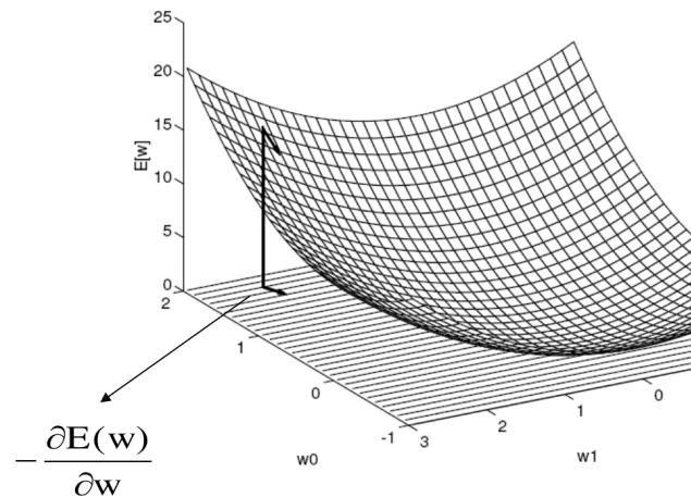
Figura 5.7: La superficie d'errore di un modello lineare con due pesi: ogni punto del piano (w_0, w_1) è un'ipotesi.
