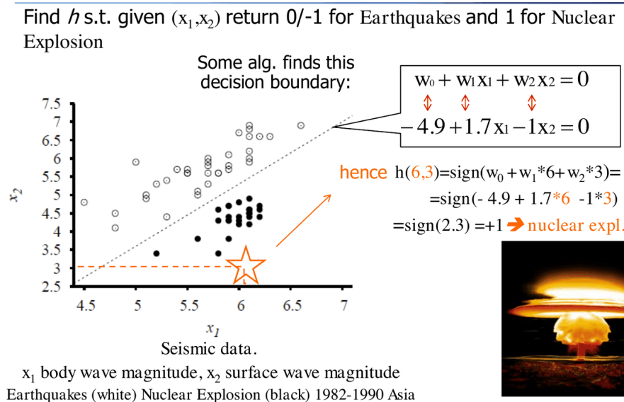
Figura 5.3: Classificazione di dati sismici con un confine di decisione lineare.
