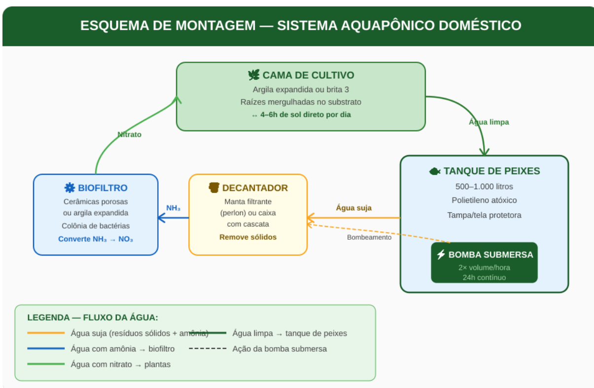
Figura 2 — Esquema de montagem: fluxo completo da água entre os componentes
