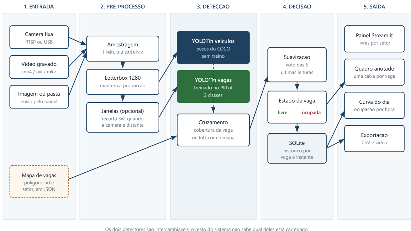
Figura 1. Arquitetura do Baliza. A faixa 3 é o núcleo de visão computacional, com os dois detectores que a seção 7 compara; a faixa 4 é o que impede o painel de piscar entre livre e ocupada a cada quadro.
