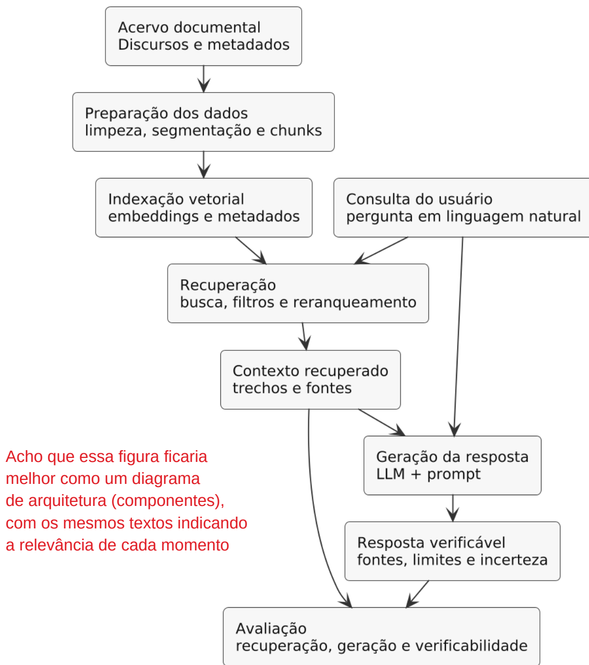
Figura 1: Componentes de um pipeline RAG relevantes para a avaliação de recuperação, geração e verificabilidade
