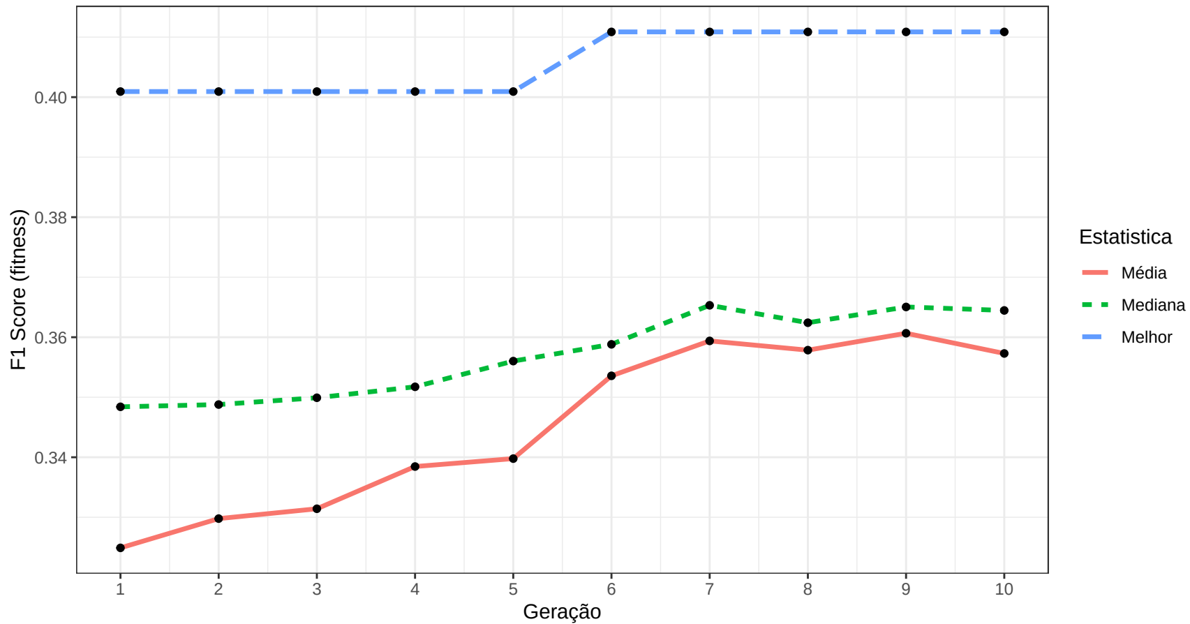
GA – Evolução F1 | Linear | Oliveira 2015 Sim6
