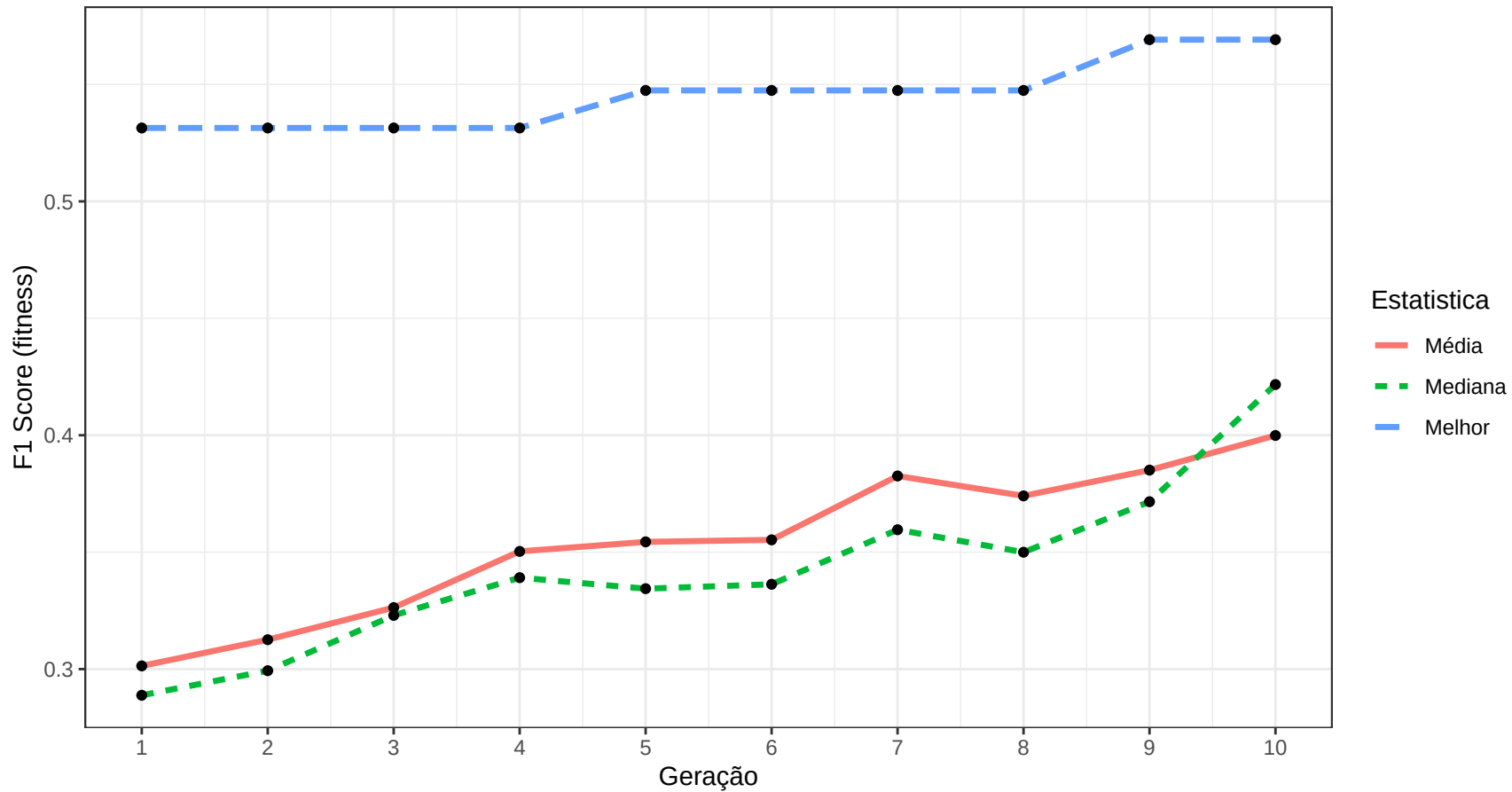
GA – Evolução F1 | Radial_0.1 | Oliveira 2015 Sim6
