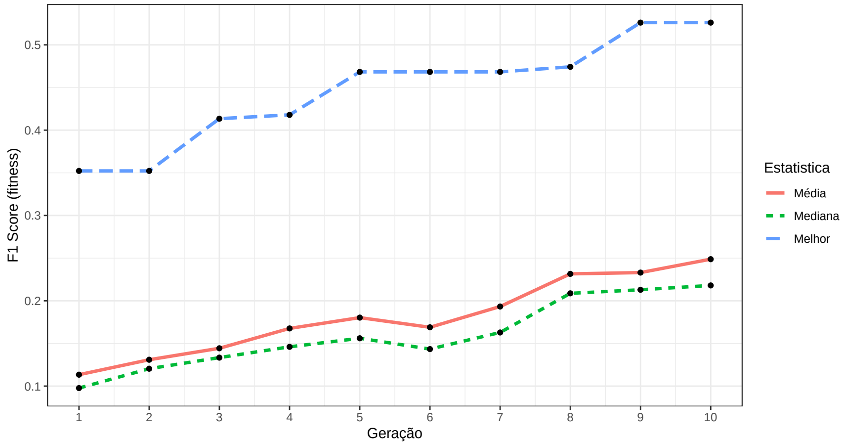
GA – Evolução F1 | Radial_1 | Oliveira 2015 Sim6
