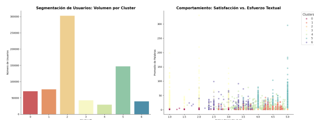
Figura 7. Segmentación de usuarios: volumen por clúster y comportamiento (satisfacción vs. esfuerzo textual).
