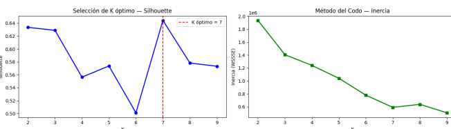
Figura 6. Selección de k : coeficiente de silueta (izq.) y método del codo sobre la inercia/WSSSE (der.). El máximo de silueta se alcanza en k = 7 .
