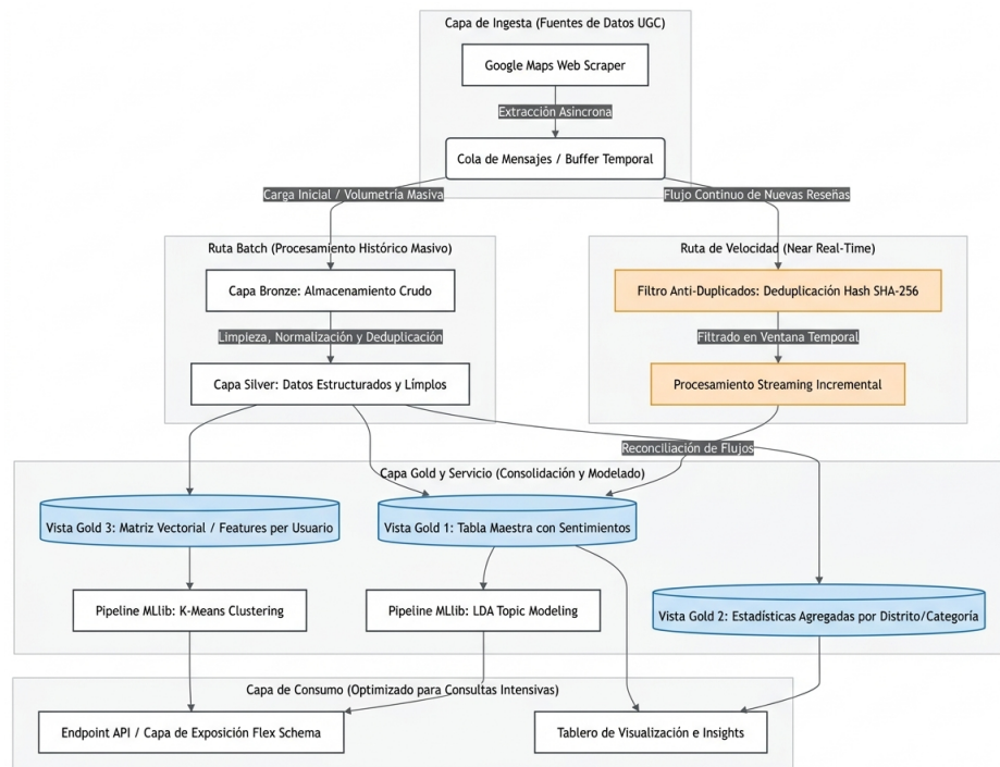
Figura 2. Arquitectura de componentes lógicos : separación de rutas batch/streaming , consolidación medallón, vistas Gold, modelamiento con MLlib y consumo por tablero o API.
