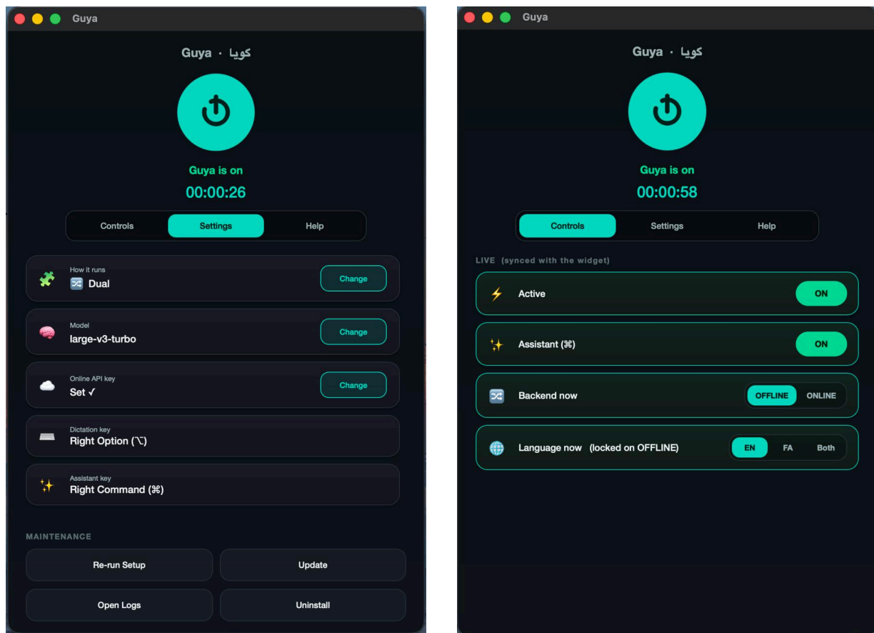
شکل ۵.۲. پنل کنترل در حالت دوگانه: زبانه Controls با کلید زنده پشتیبان و زبانی که در حالت OFFLINE قفل شده، و زبانه Settings با حالت، مدل، کلید آنلاین و دو کلید میانبر.
