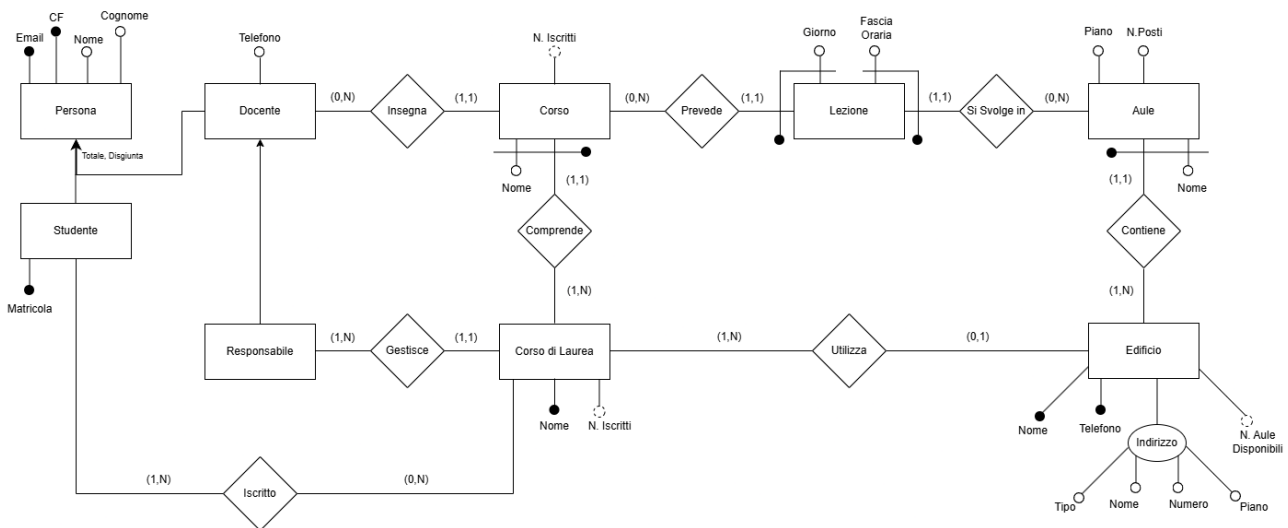
Figura 1: Schema E-R del sistema per la gestione del calendario delle lezioni
