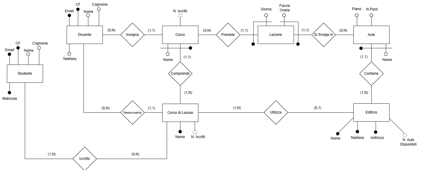
Figura 2: Schema ER privo di generalizzazioni
