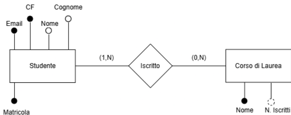
Figura 3: Sotto-schema E-R per l'analisi delle ridondanze sul attributo n° iscritti
