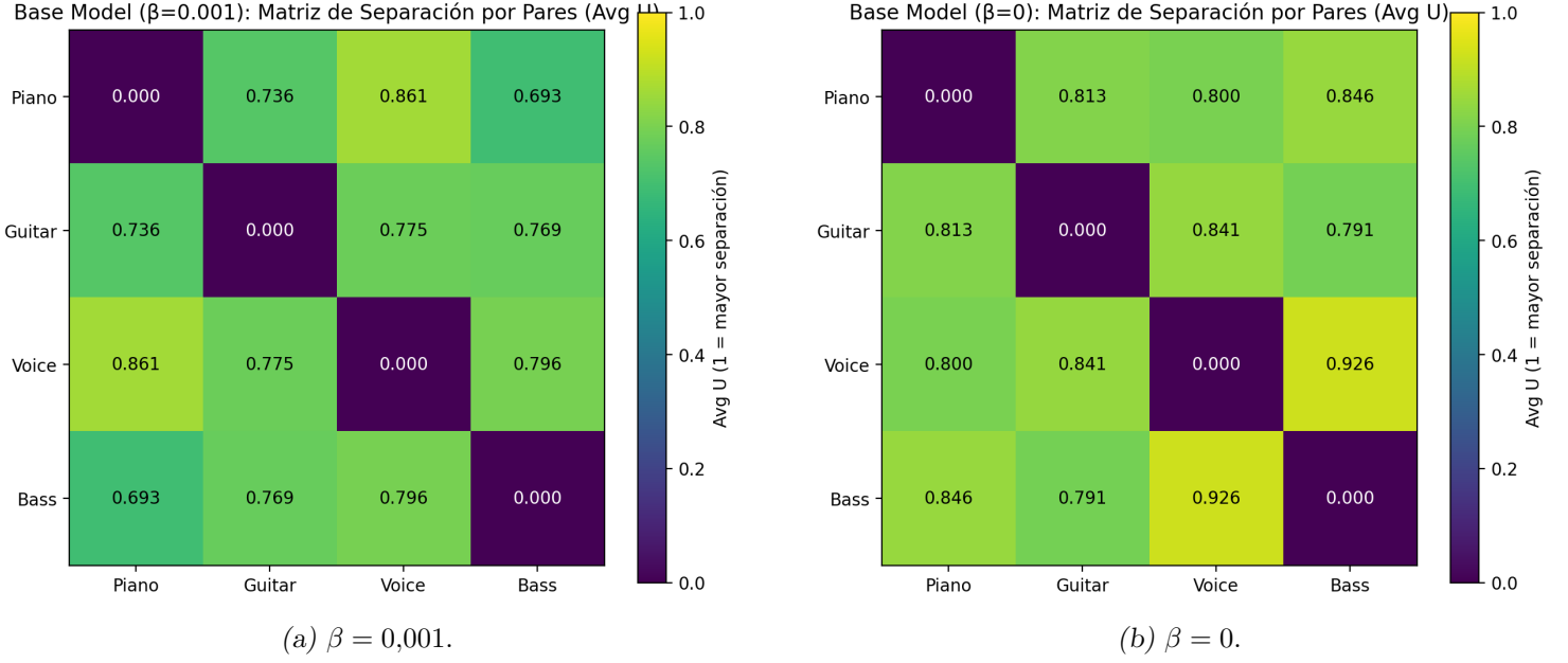
Fig. 3.7: Matriz de separación entre clusters de instrumentos en la proyección UMAP.
