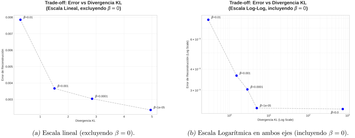
Fig. 3.5: Curva de compromiso entre error de reconstrucción y divergencia KL para la selección del hiperparámetro \beta .
