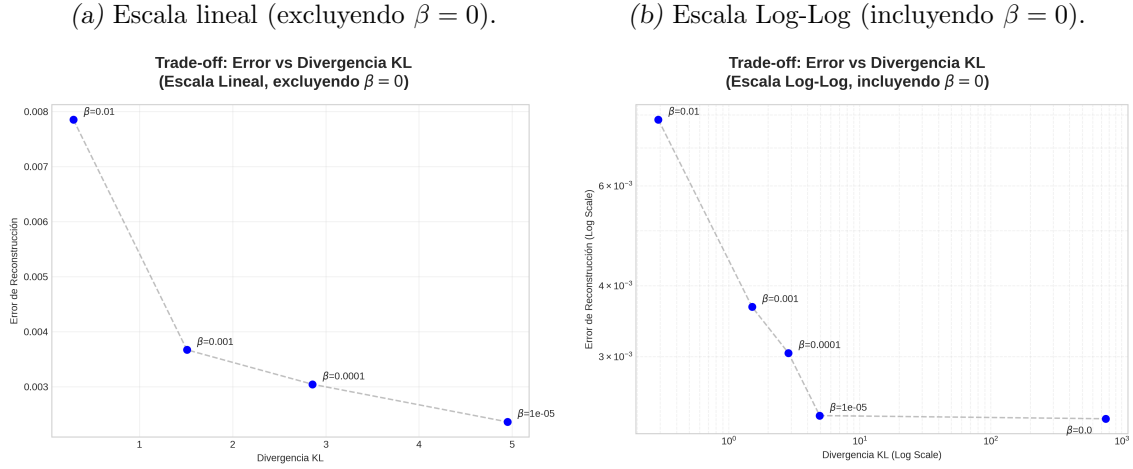
Fig. 3.2: Frontera de Pareto para la selección del hiperparámetro \beta .
