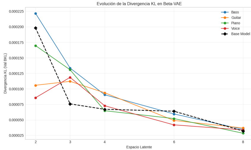
Fig. 3.4: Divergencia KL vs Dimensión de espacio latente, \beta = 0,001
