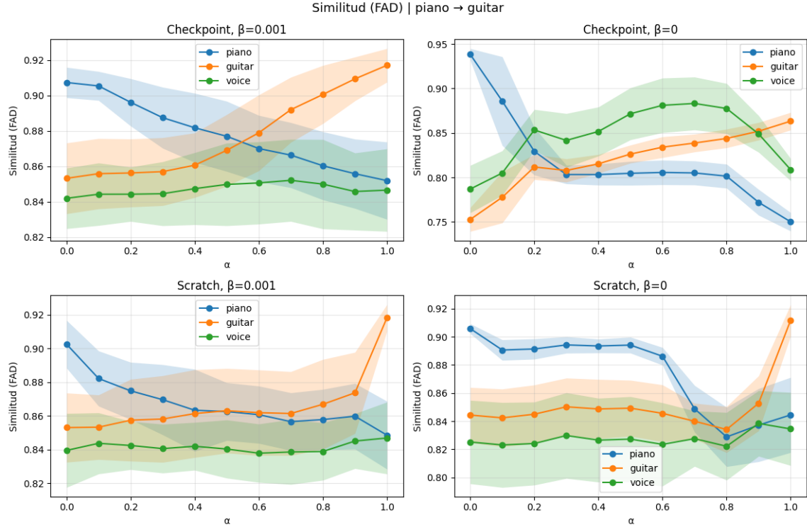
Fig. 3.14: Transición cruzada de piano a guitarra. Comparación entre orígenes ( Checkpoint vs. Scratch ) y regularización ( \beta ). La voz actúa como instrumento testigo.
