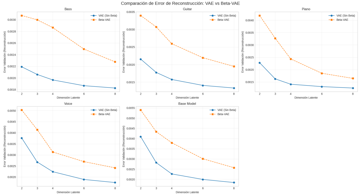
Fig. 3.5: Desglose: Error de Reconstrucción (MSE) por modelo
