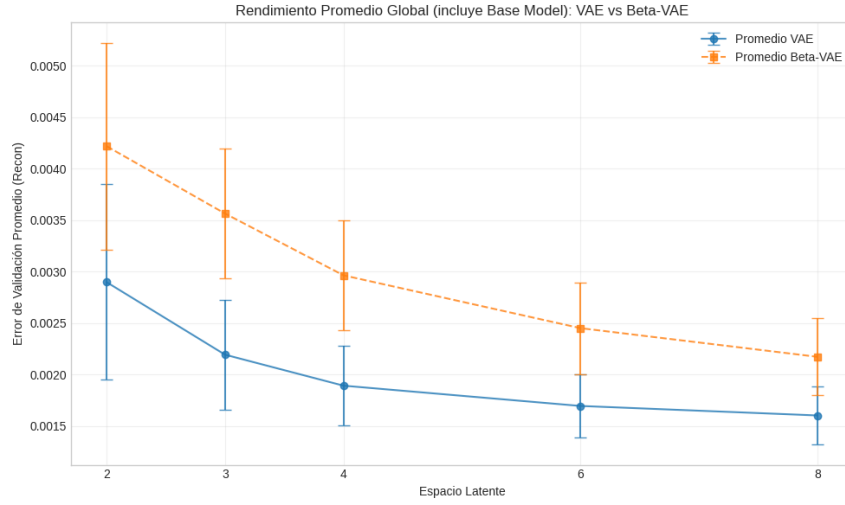
Fig. 3.3: Error de Reconstrucción promedio general
