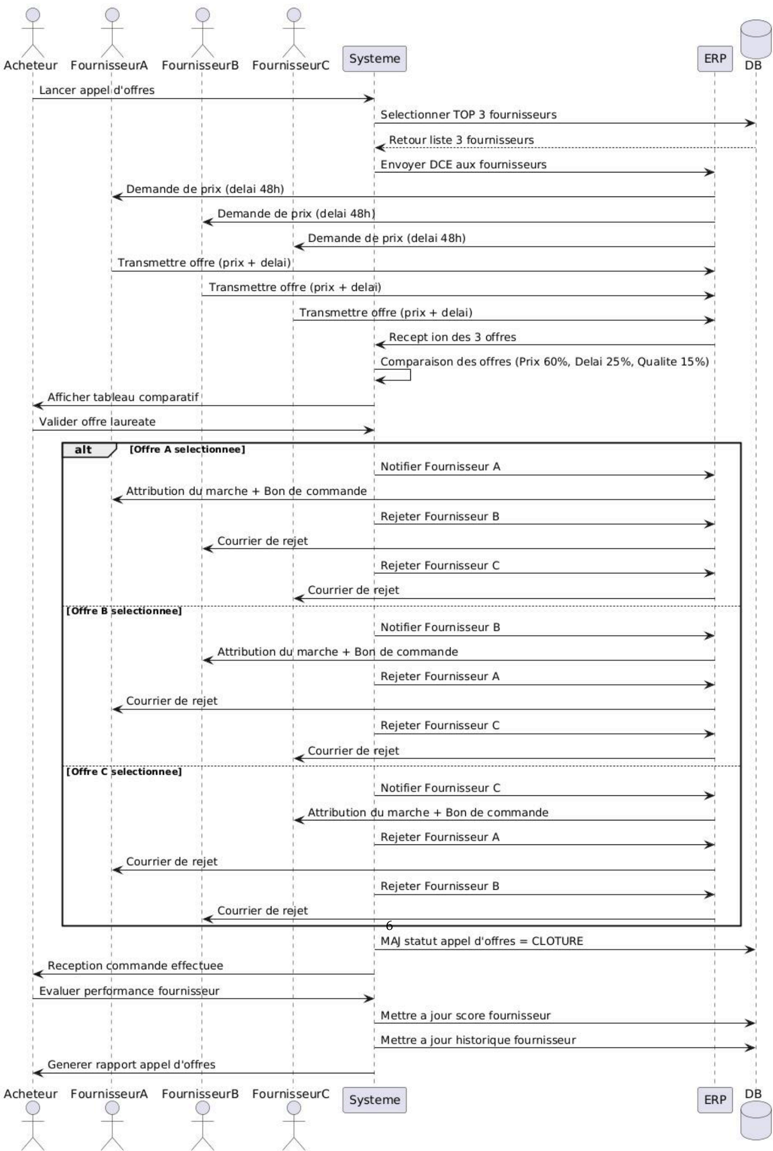
Diagramme de Séquence — Appel d’offres et gestion fournisseurs
