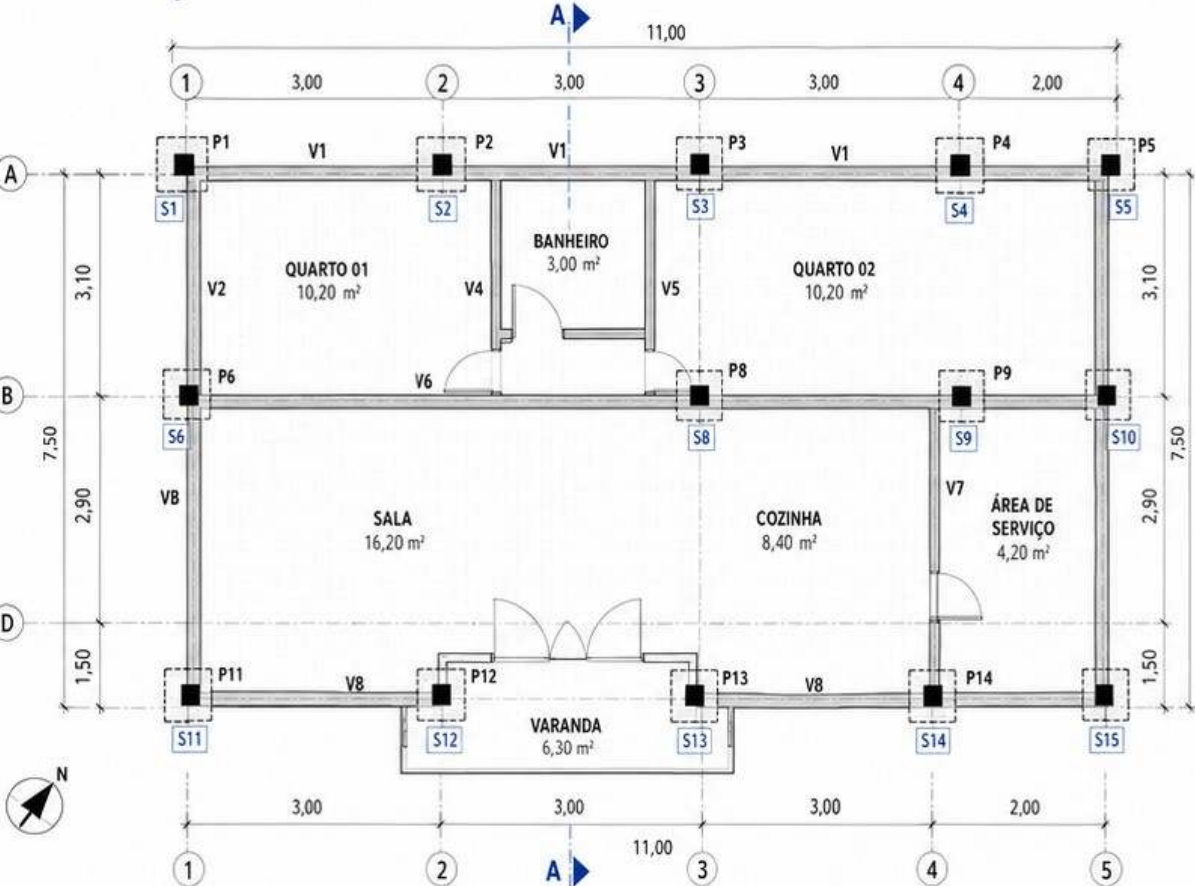
PLANTA DE LANÇAMENTO ESTRUTURAL ESCALA 1:75 (INDICADA) COTAS EM METROS DIMENSÕES CONCEITUAIS – A VALIDAR
