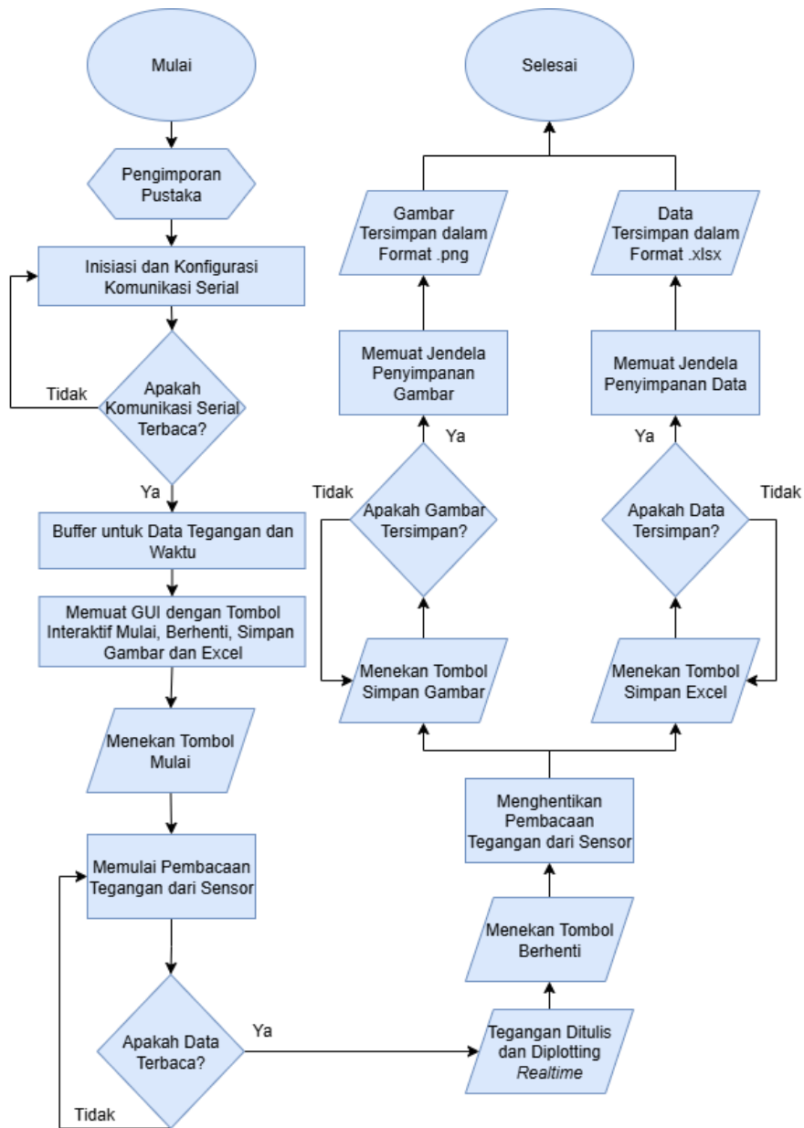
Gambar 3.7. Diagram Alir Pemrograman Perangkat Lunak Python
