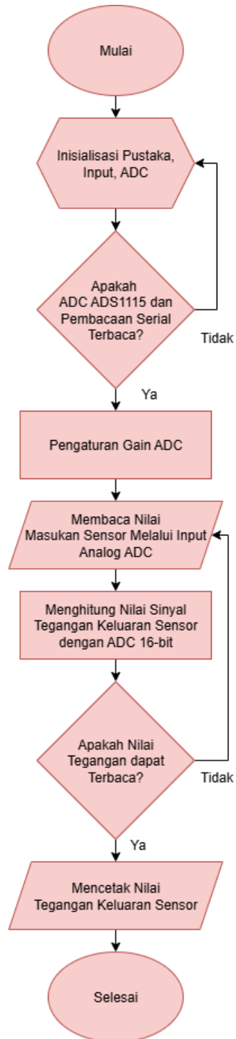
Gambar 3.5. Diagram Alir Pemrograman Perangkat Lunak Mikrokontroler
