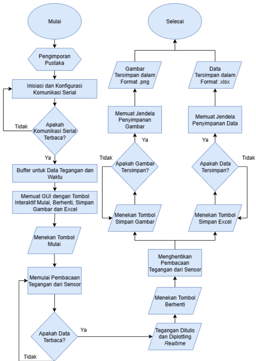
Gambar 3.6. Diagram Alir Pemrograman Perangkat Lunak Python
