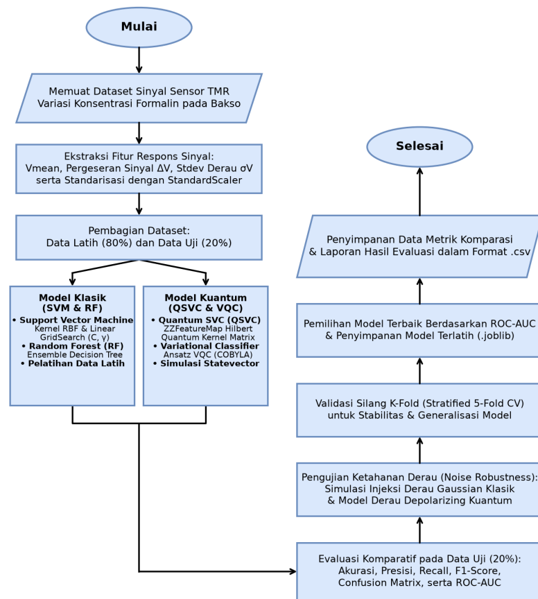
Gambar 3.7. Diagram Alir Pembuatan, Pelatihan, dan Komparasi Model Klasifikasi (Model Klasik: SVM, RF vs. Model Kuantum: QSVC, VQC)
