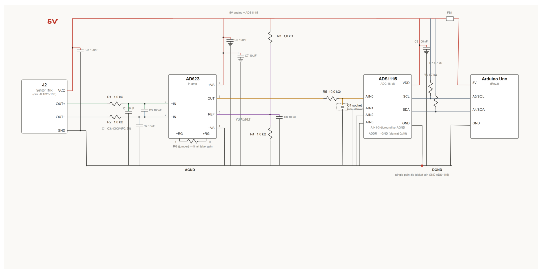
Gambar 3.4. Desain Rangkaian Perangkat Keras Instrumentasi Sensor TMR ALT023-10E
