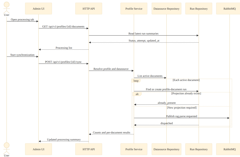
Gambar III.39: Diagram urutan sinkronisasi dokumen datasource ke profile
