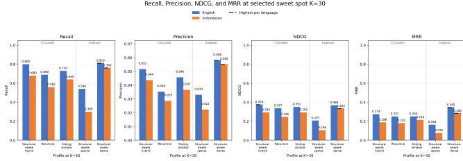
Fig. 2. Metrik seluruh konfigurasi hukum pada K = 30 .
