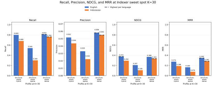
Fig. 1. Metrik indexer User Manual pada K = 30 .
