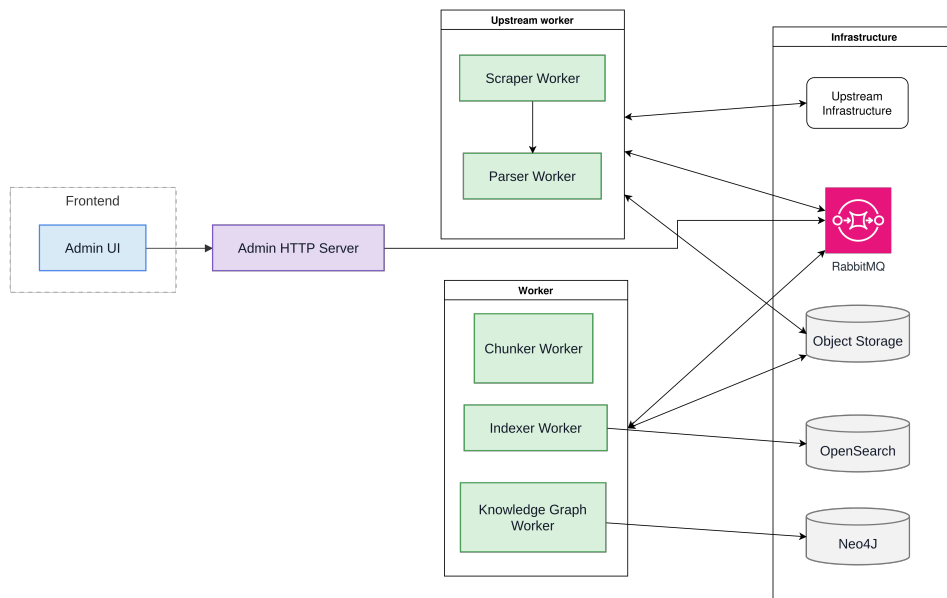
Gambar III.11: Arsitektur sistem service pemrosesan offline Omni-RAG
