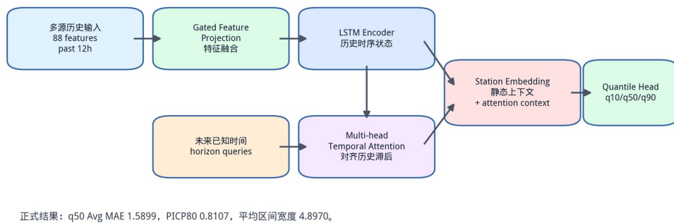
图4-3 TFT-style 分位数预测模块结构
