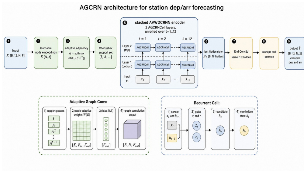
图 4-1 AGCRN 基线模型总体结构
