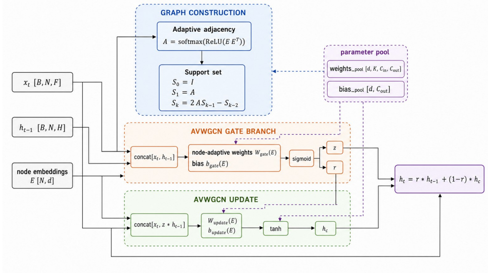
图 4-2 AGCRN 单元与自适应图卷积细节
