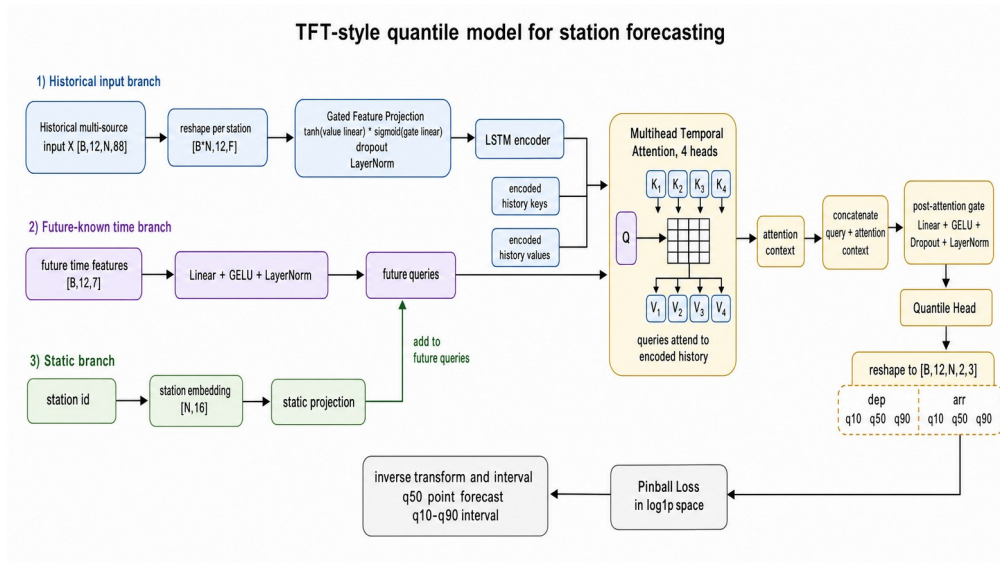
图 4-5 TFT-style 分位数预测模块总体结构
