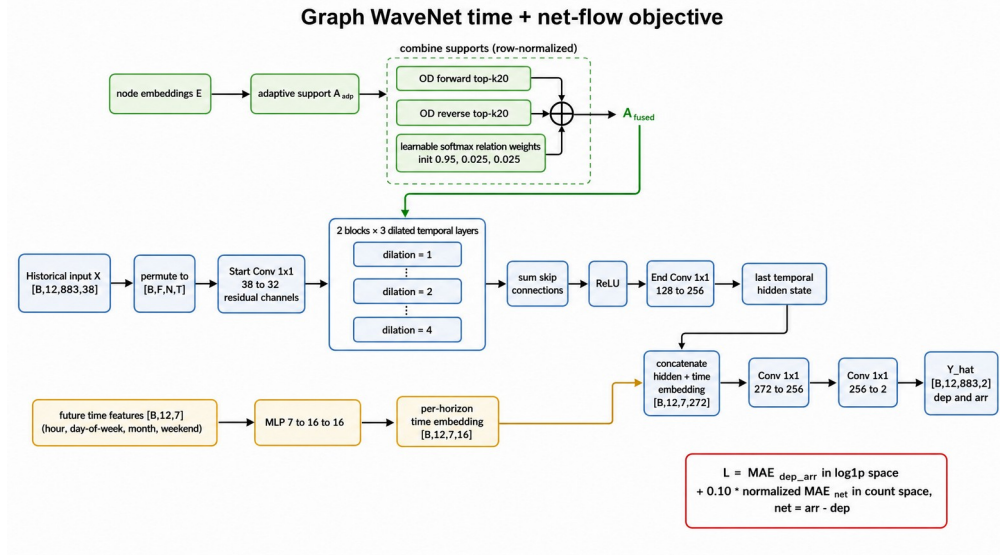
图 4-3 Graph WaveNet（目标时间特征与净流量辅助损失）总体结构
