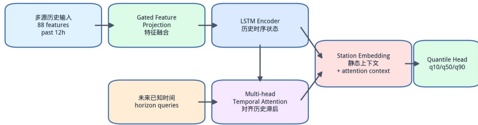
图4-3 TFT-style 分位数预测模块结构
