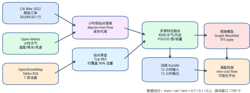
图3-1 数据处理与特征工程流程
