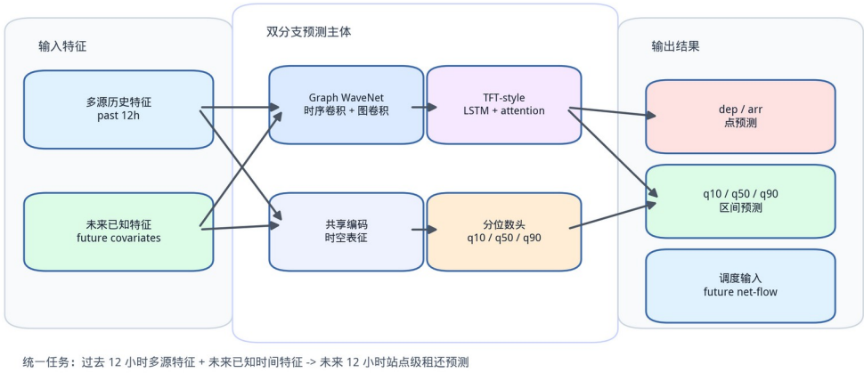
图 4-1 预测模型总体结构
