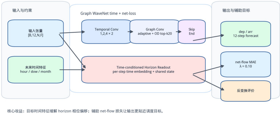
图 4-2 Graph WaveNet（目标时间特征与净流量辅助损失）模型结构
