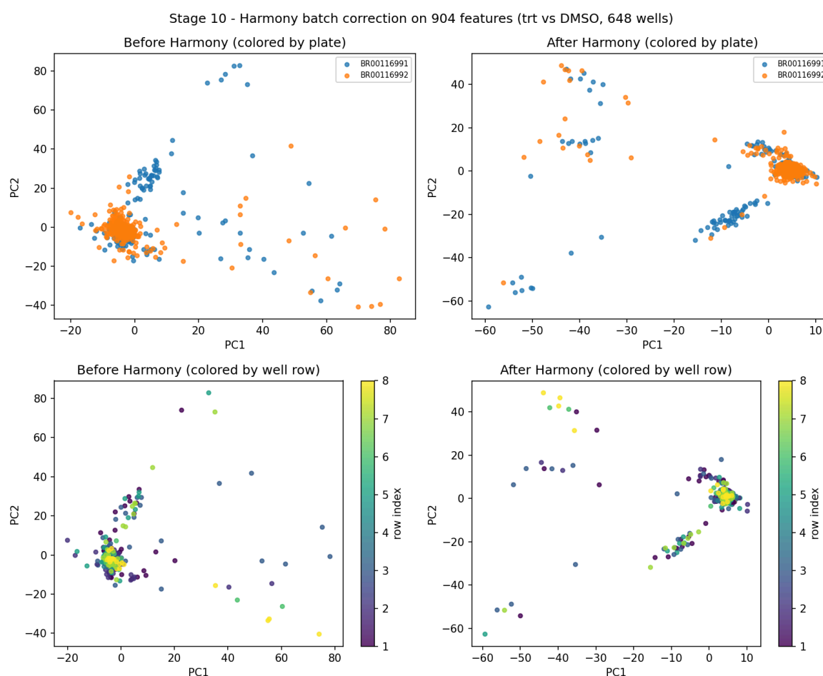
Harmony batch correction PCA
